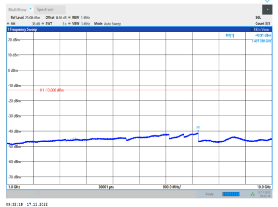
EGPRS850-190-8-1000~10000MHz
