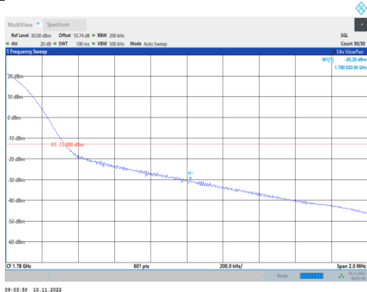
Band66-20MHz-QPSK-132572-1RB#99
