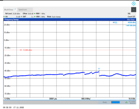
EGPRS850-251-8-1000~10000MHz
