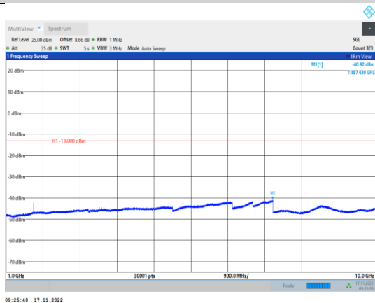
GPRS850-128-3-1000~10000MHz
