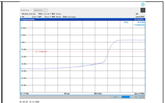
Band66-10MHz-QPSK-132022-50RB#0
