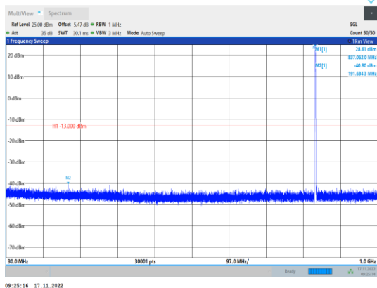
GPRS850-128-3-30~1000MHz
