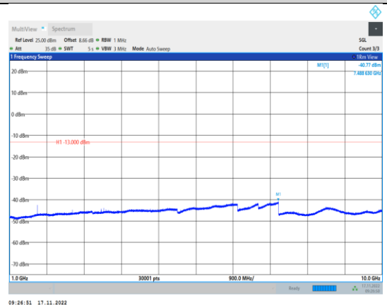
GPRS850-251-3-1000~10000MHz
