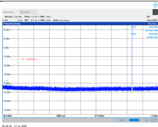
GPRS850-190-3-30~1000MHz
