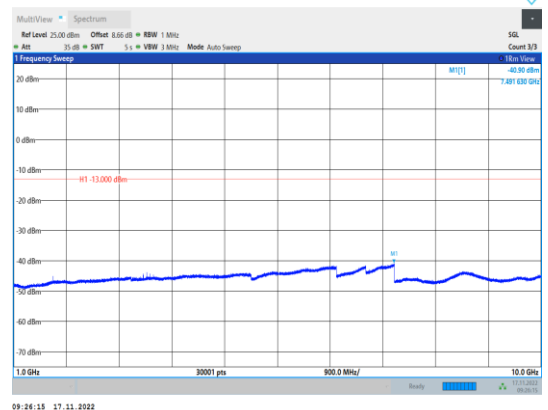
GPRS850-190-3-1000~10000MHz
