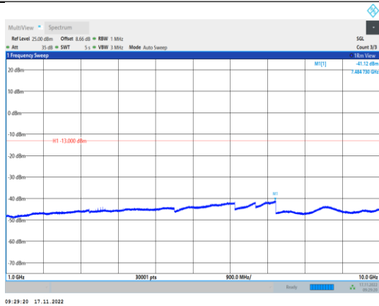
EGPRS850-128-8-1000~10000MHz
