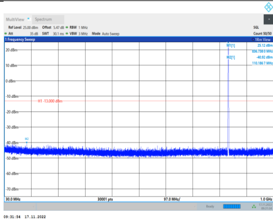
EGPRS850-190-8-30~1000MHz
