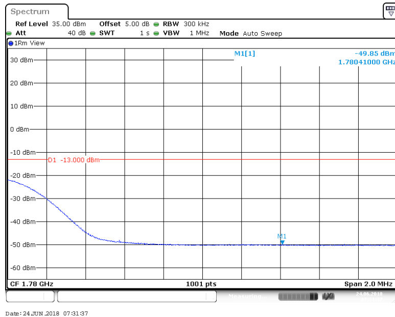
BAND 66_20MHz_QPSK_132572_1RB#99
