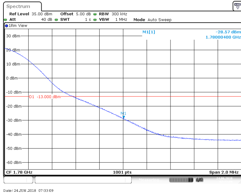
BAND 66_20MHz_QPSK_132572_100RB#0
