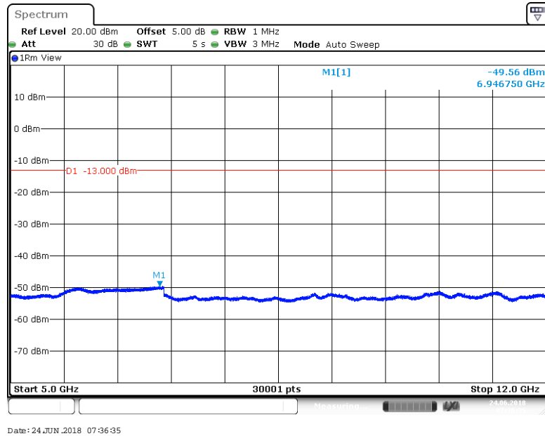
BAND 66_20MHz_QPSK_132072_1RB#0
