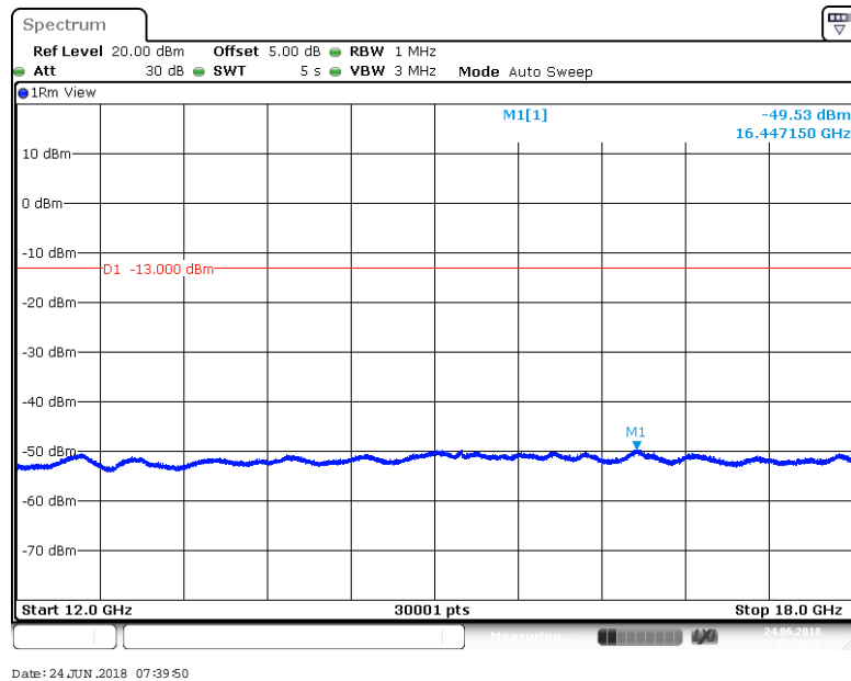
BAND 66_20MHz_QPSK_132572_1RB#0
