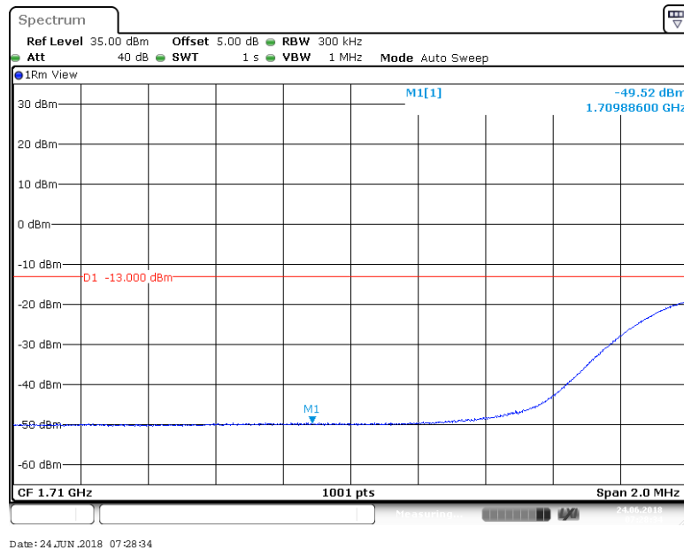
BAND 66_20MHz_QPSK_132072_100RB#0
