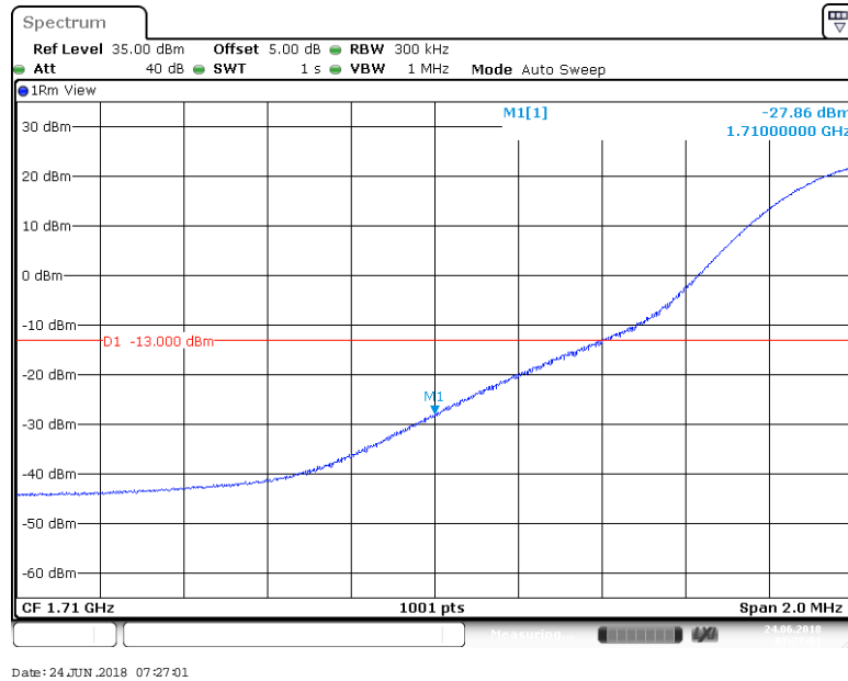
BAND 66_20MHz_QPSK_132072_1RB#99
