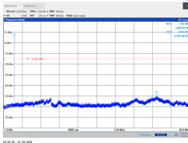
3DH5 Ant1 2480 1000~26500
