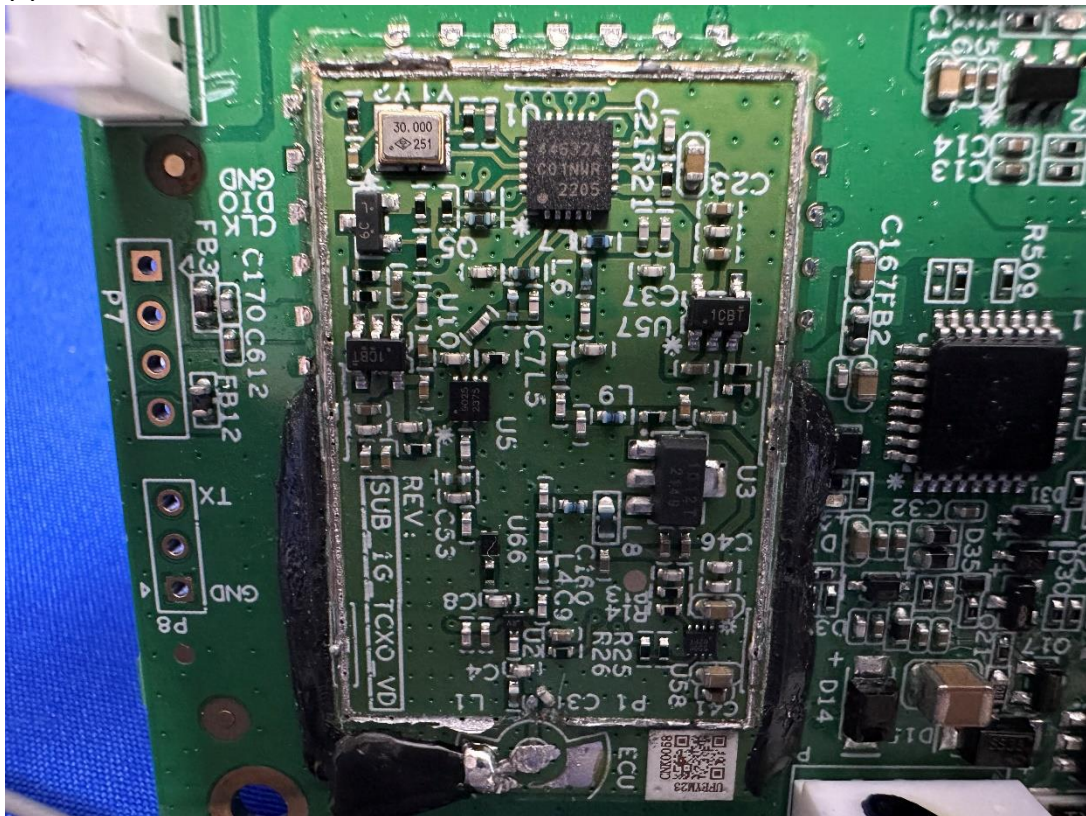
(9) EUT Photo
