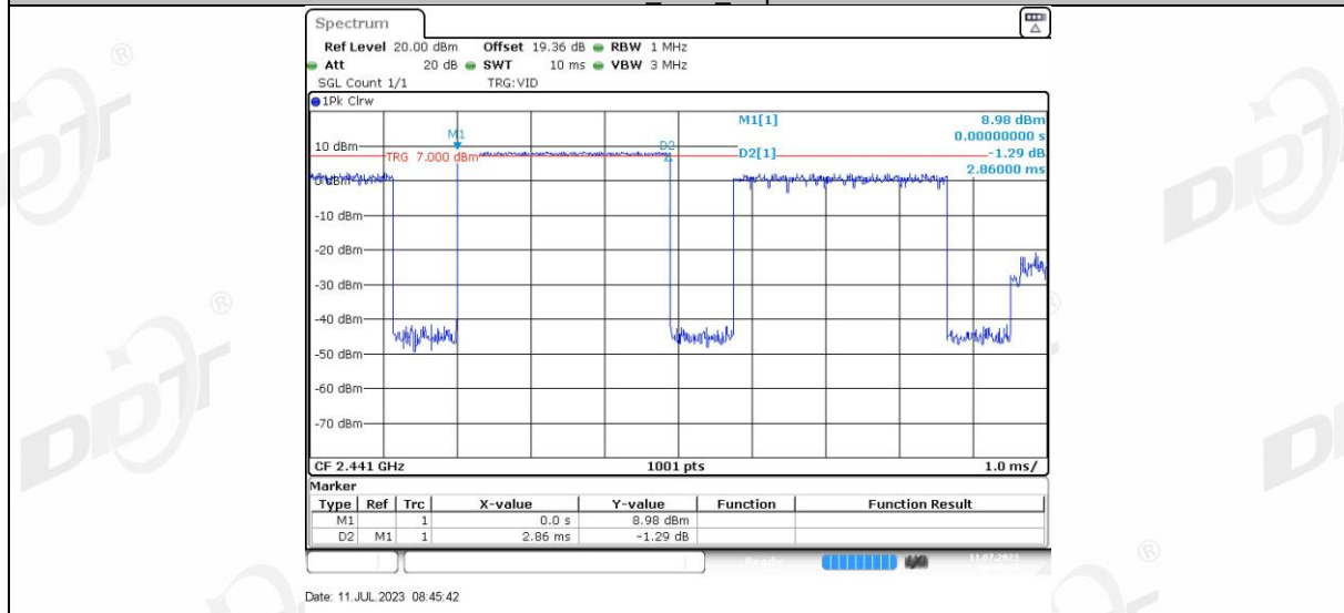
2DH5_Ant1_Hop
