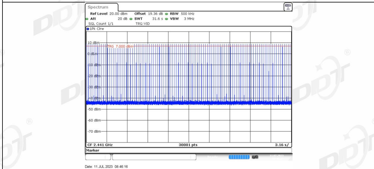
3DH1_Ant1_Hop
