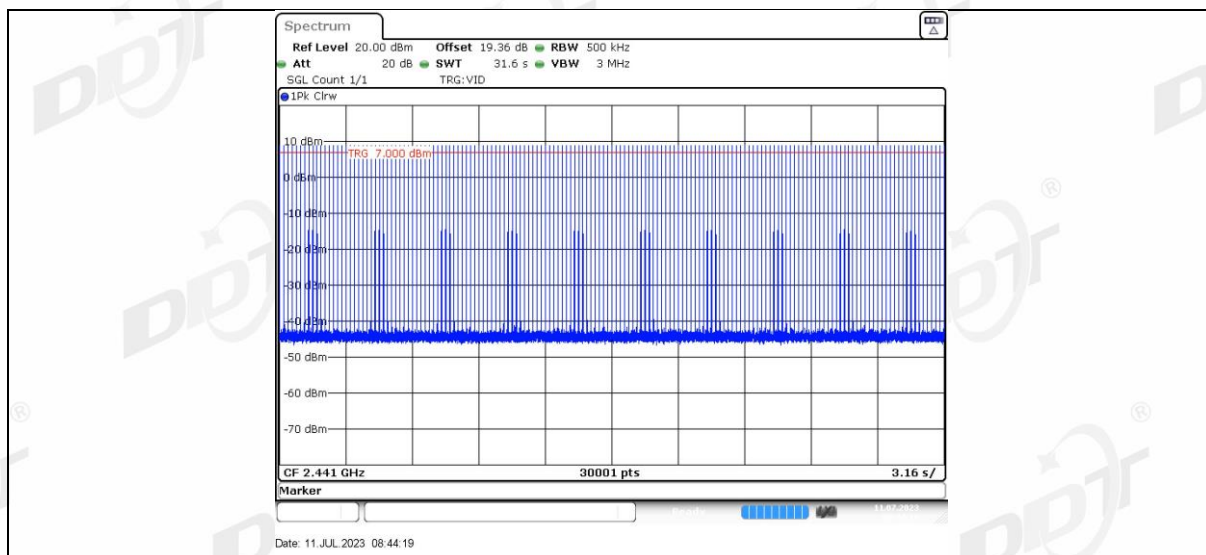
DH5_Ant1_Hop
