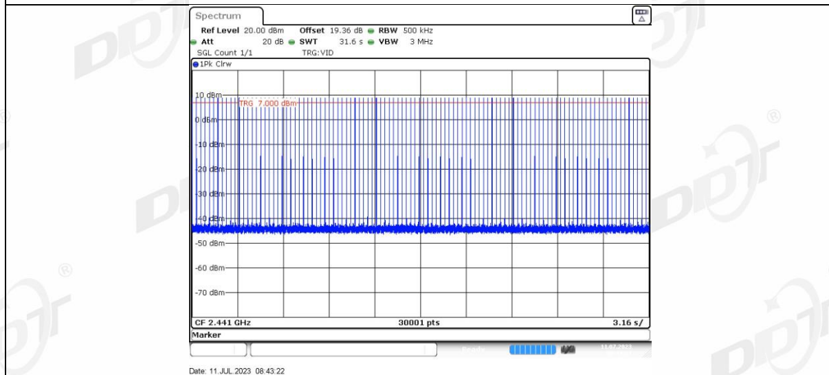
2DH1_Ant1_Hop
