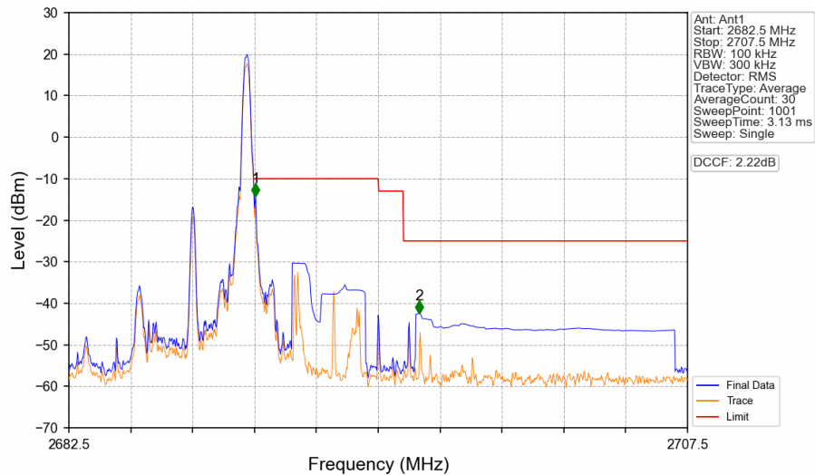
Band41_5MHz_QPSK_HCH_2687.5MHz_RB_1_24_NTNV
