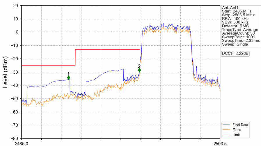
Band41_5MHz_QPSK_LCH_2498.5MHz_RB_25_0_NTNV
