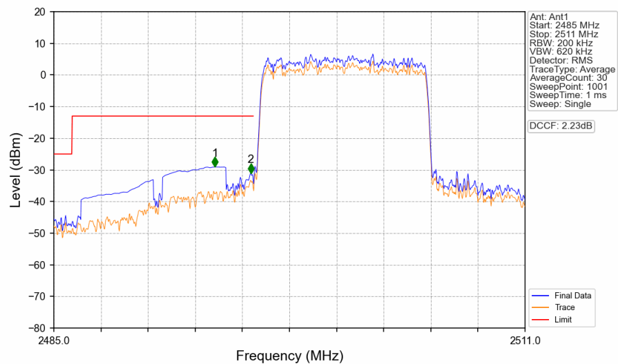
Band41_10MHz_16QAM_LCH_2501MHz_RB_50_0_NTNV
