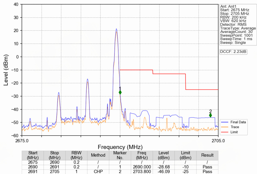
Band41_10MHz_16QAM_HCH_2685MHz_RB_1_49_NTNV
