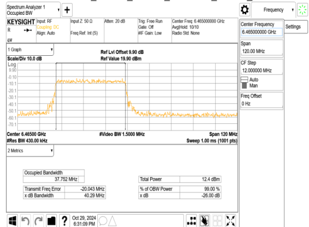
802.11ax_80MHz_ChainB_6465MHz_RU484_66
