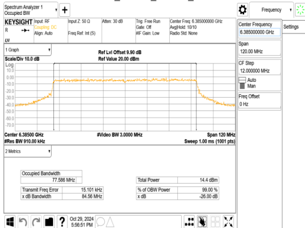
802.11ax_80MHz_ChainB_6385MHz_RU484_66
