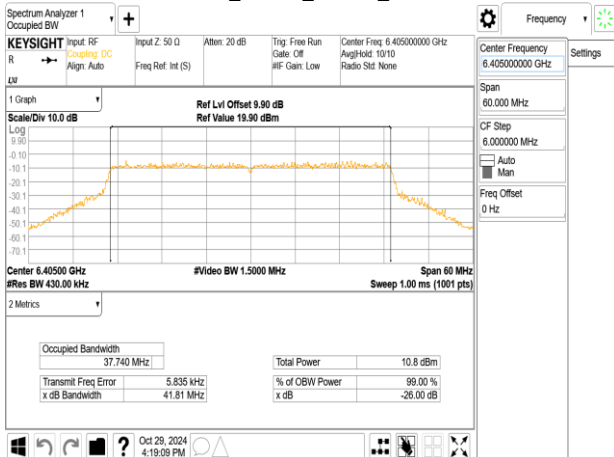
802.11ax_40MHz_ChainB_6405MHz
