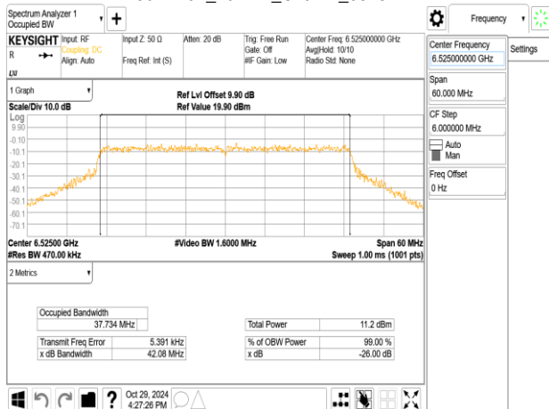
802.11ax_40MHz_ChainB_6525MHz
