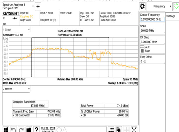
802.11ax_20MHz_ChainB_6895MHz_RU26_0
