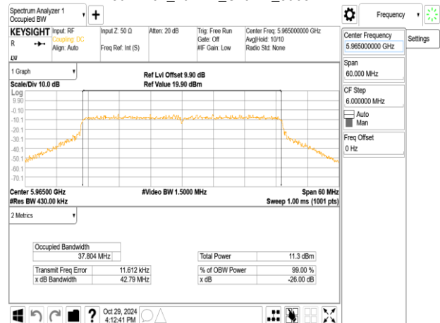
802.11ax_40MHz_ChainB_5965MHz
