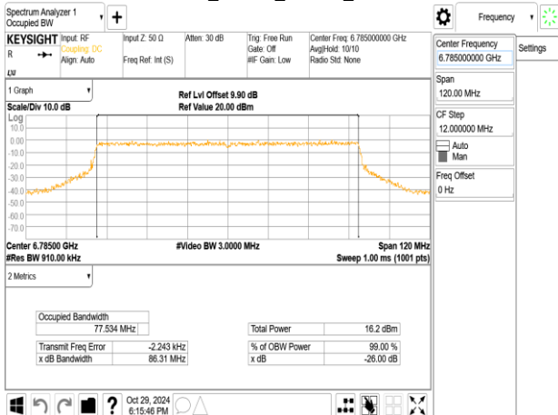
802.11ax_80MHz_ChainA_6785MHz
