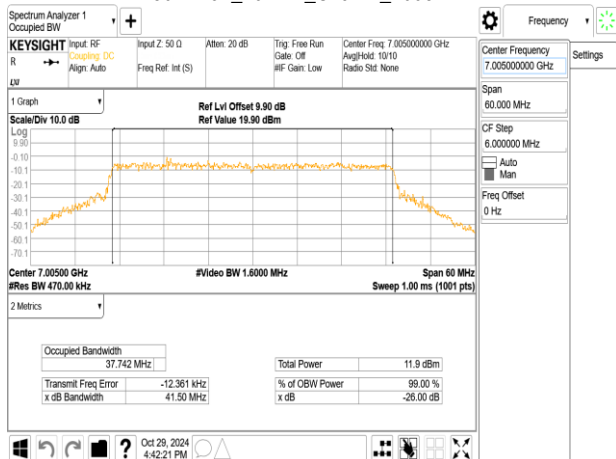
802.11ax_40MHz_ChainA_7005MHz
