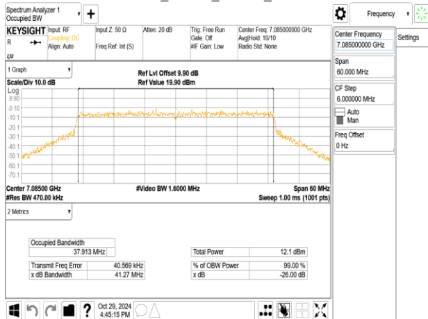
802.11ax_40MHz_ChainB_7085MHz_RU242_62
