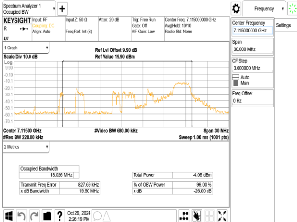
802.11ax_20MHz_ChainB_7115MHz_RU52_40
