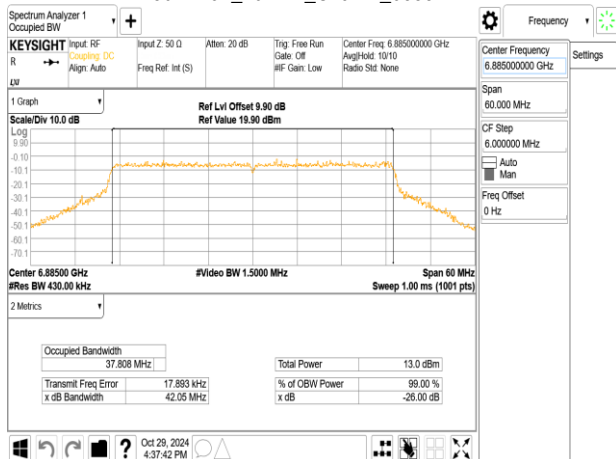
802.11ax_40MHz_ChainB_6885MHz
