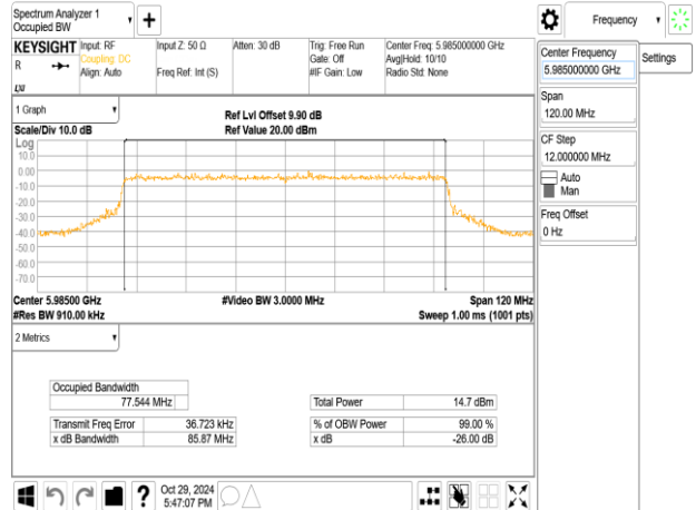
802.11ax_80MHz_ChainB_5985MHz_RU484_65
