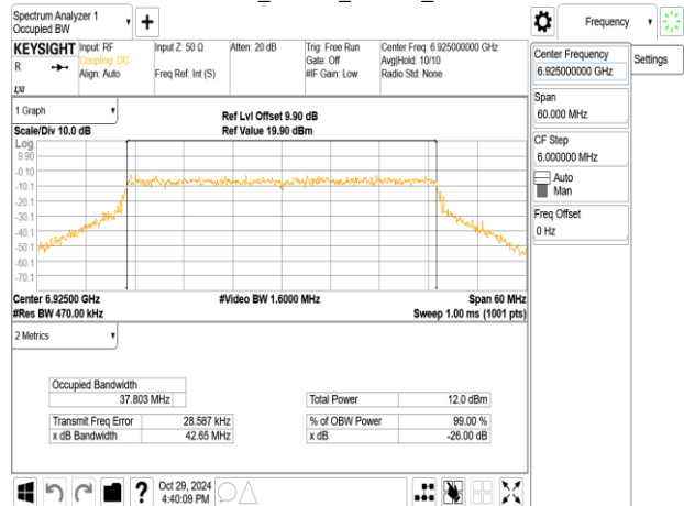
802.11ax_40MHz_ChainB_6925MHz_RU242_61
