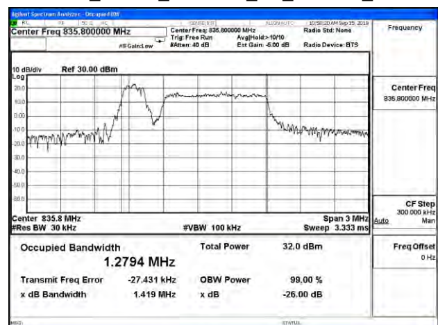
Cat M1_Band 5_CH20525_3M_16-QAM_5RB1
