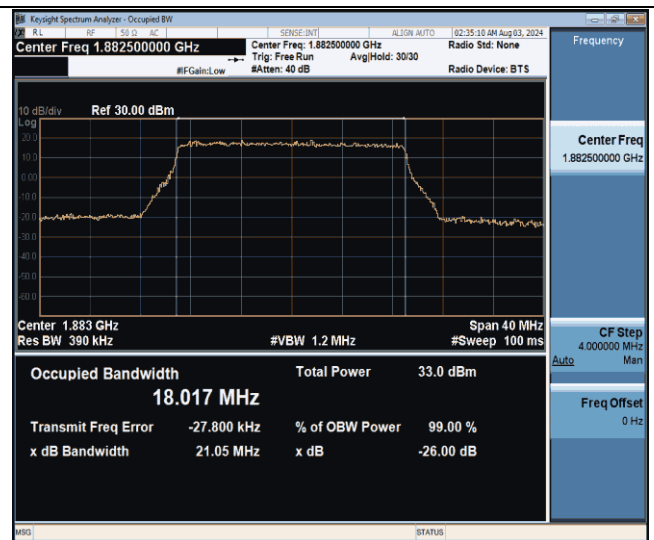
Band25-20MHz-QPSK-26365-100RB#0-PASS
