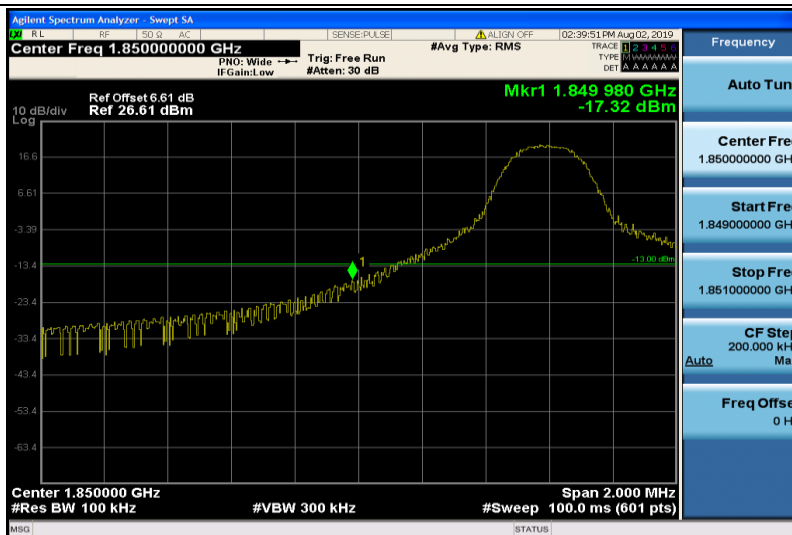
Band2-10MHz-QPSK-18650-1RB#0
