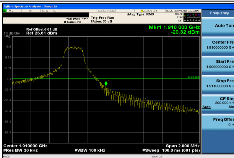
Band2-3MHz-QPSK-19185-1RB#14
