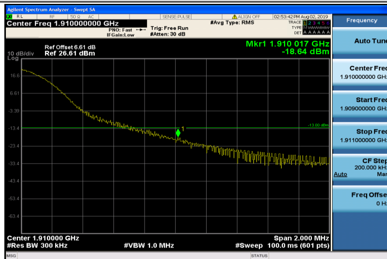
Band2-20MHz-16QAM-19100-1RB#99
