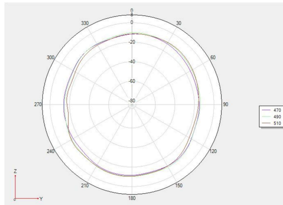
Phi 90 2D图
