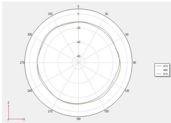
Phi 0 2D图
