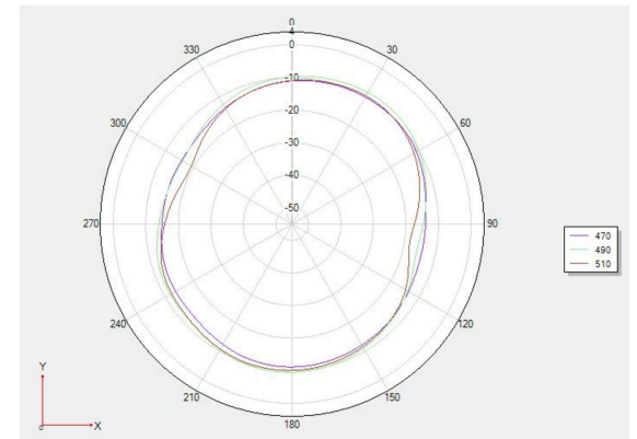
Theta 90 2D图
