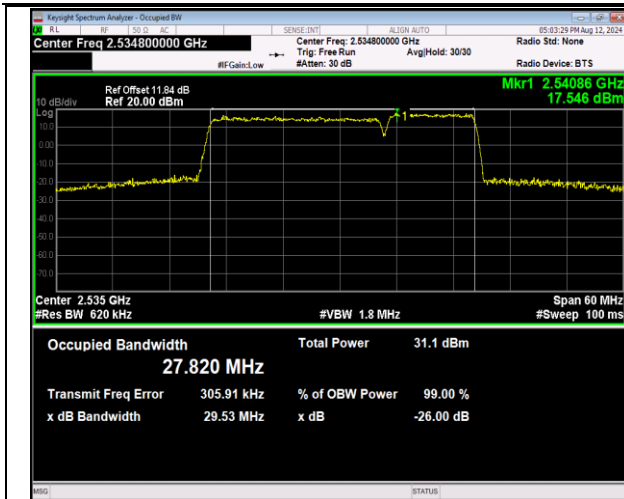
7-7-20MHz-10MHz-QPSK-QPSK-21051-21195-100RB#0-50RB#0-PASS
