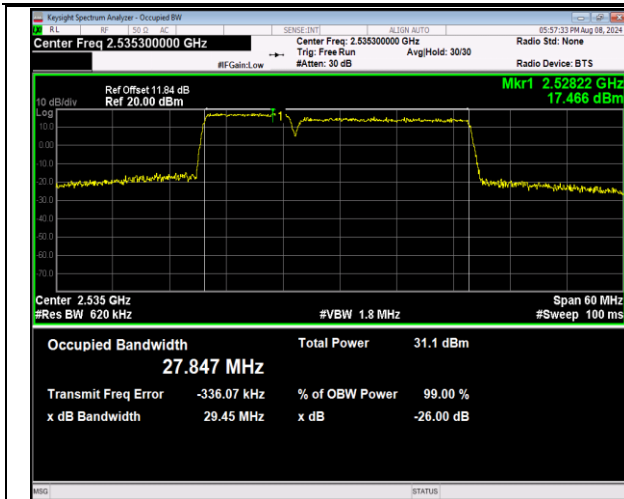
7-7-10MHz-20MHz-QPSK-QPSK-21006-21150-50RB#0-1 00RB#0-PASS
