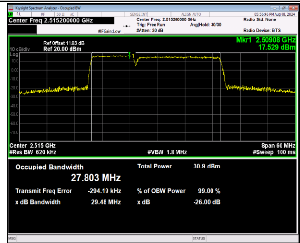
7-7-10MHz-20MHz-QPSK-QPSK-20805-20949-50RB#0- 100RB#0-PASS
