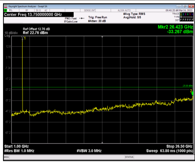
Band7-5MHz-16QAM-21425-1RB#0-Range2:1000~26 500MHz
