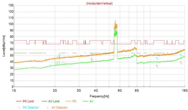
11N_20M_5720
