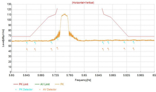
11N_20M_5745
