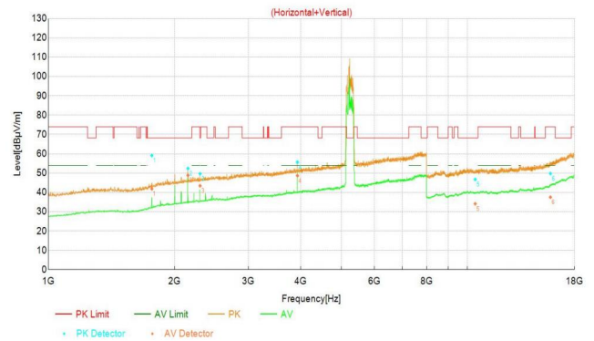
11N_20M_5300
