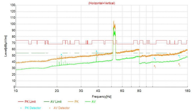
11N_20M_5240
