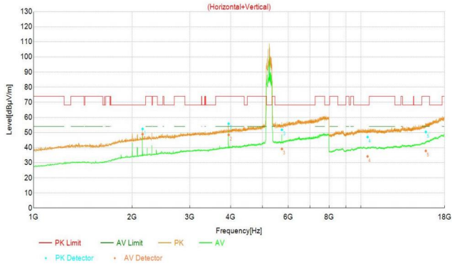
11N_20M_5320
