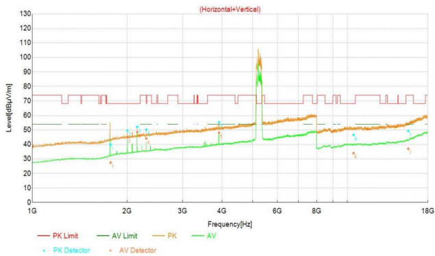
11N_20M_5260
