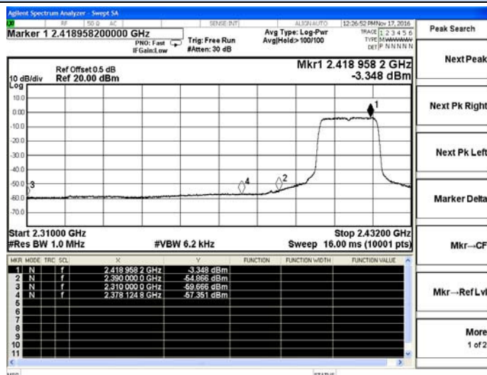
802.11n(HT20)-Low channel(Average)
