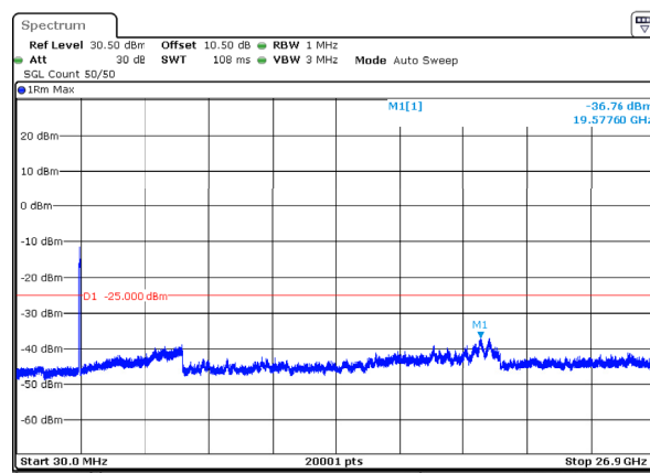
n41_80MHz_30kHz_2649.99MHz_DFT-s-OFDM QPSK_RB216@0 -36.76dBm
