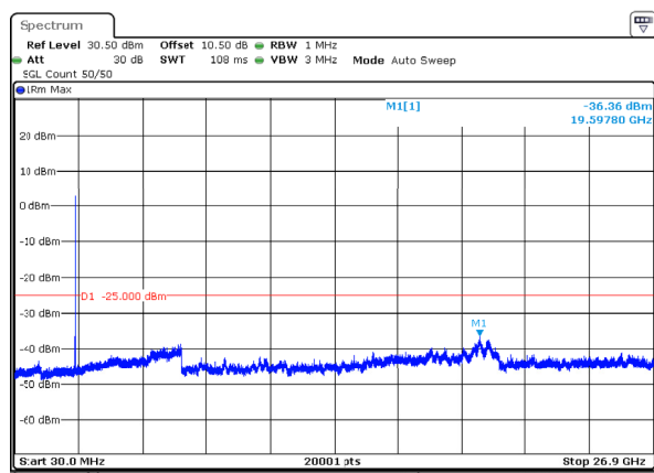
n41_80MHz_30kHz_2536.02MHz_DFT-s-OFDM QPSK_RB1@216 -36.36dBm
