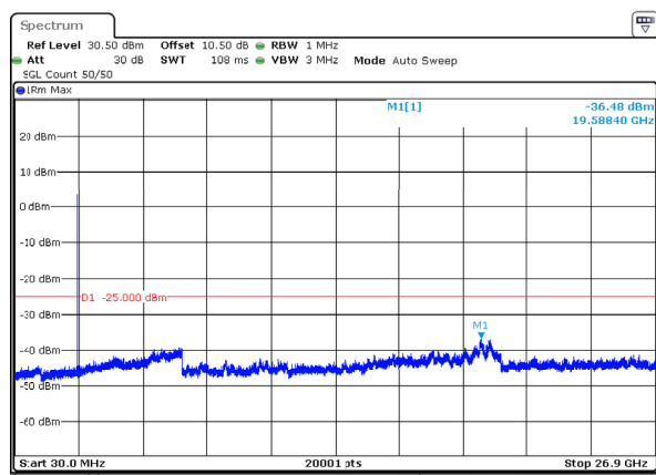
n41_50MHz_30kHz_2664.99MHz_DFT-s-OFDM QPSK_RB1@0 -36.48dBm
