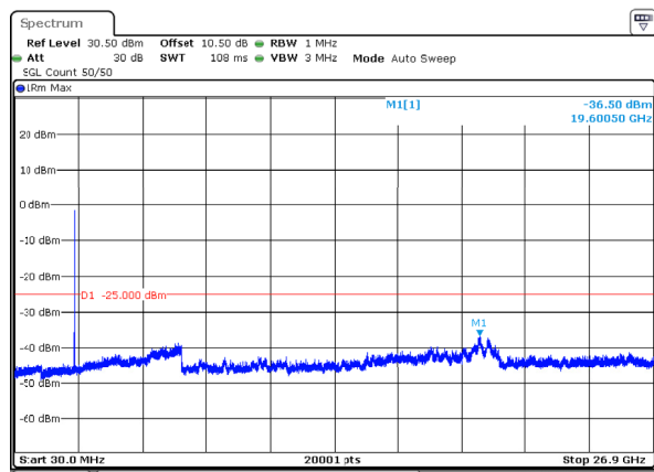
n41_40MHz_30kHz_2516.01MHz_DFT-s-OFDM QPSK_RB1@105 -36.50dBm
