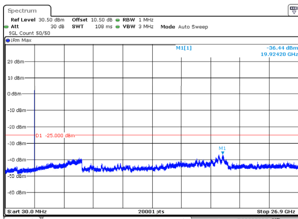
n41_15MHz_30kHz_2682.48MHz_DFT-s-OFDM QPSK_RB1@37 -36.44dBm
