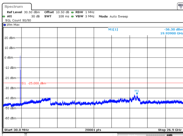
n41_60MHz_30kHz_2592.99MHz_DFT-s-OFDM QPSK_RB1@0 -36.30dBm
