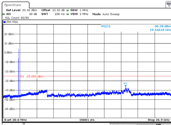
n41_20MHz_30kHz_2506.02MHz_DFT-s-OFDM QPSK_RB1@0 -36.28dBm
