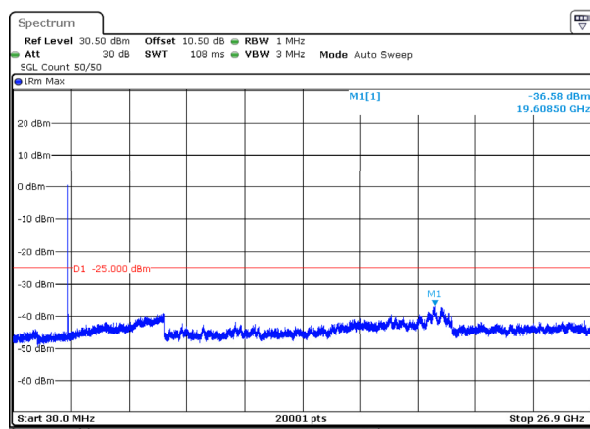
n41_80MHz_30kHz_2592.99MHz_DFT-s-OFDM QPSK_RB1@0 -36.58dBm
