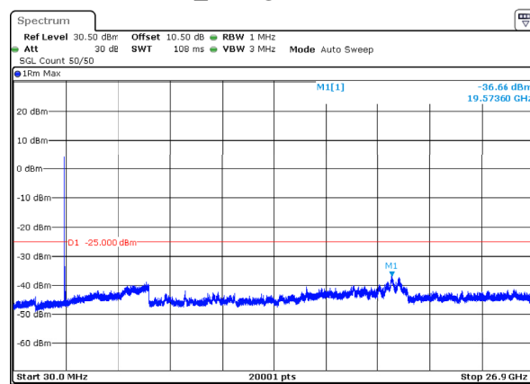
n41_80MHz_30kHz_2649.99MHz_DFT-s-OFDM QPSK_RB1@0 -36.66dBm
