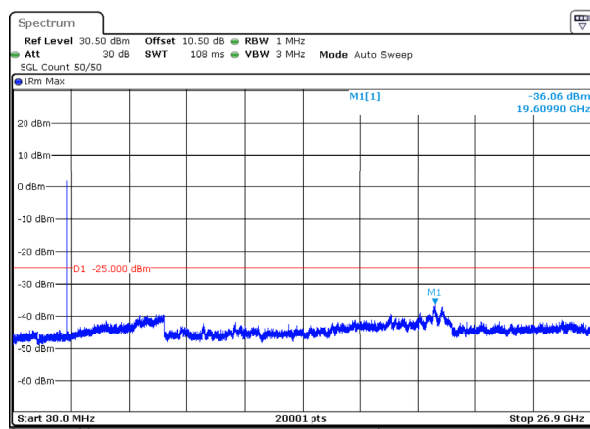
n41_30MHz_30kHz_2511MHz_DFT-s-OFDM QPSK_RB1@77 -36.06dBm
