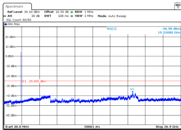
n41_30MHz_30kHz_2592.99MHz_DFT-s-OFDM QPSK_RB1@0 -36.90dBm
