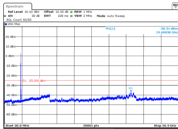
n41_80MHz_30kHz_2536.02MHz_DFT-s-OFDM QPSK_RB1@0 -36.54dBm
