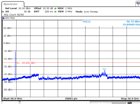
n41_60MHz_30kHz_2526MHz_DFT-s-OFDM QPSK_RB162@0 -36.73dBm
