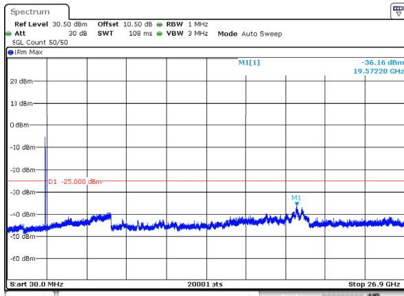
n41_15MHz_30kHz_2592.99MHz_DFT-s-OFDM QPSK_RB36@0 -36.16dBm
