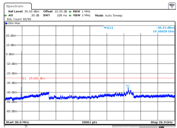
n41_60MHz_30kHz_2592.99MHz_DFT-s-OFDM QPSK_RB1@161 -36.51dBm
