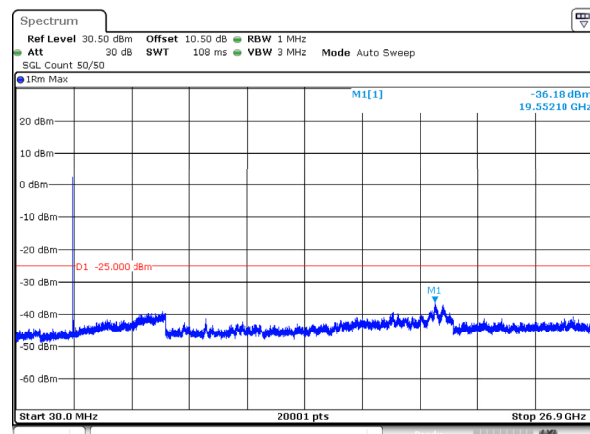
n41_40MHz_30kHz_2670MHz_DFT-s-OFDM QPSK_RB1@0 -36.18dBm
