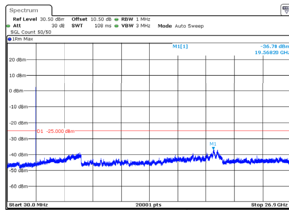
n41_20MHz_30kHz_2679.99MHz_DFT-s-OFDM QPSK_RB1@50 -36.70dBm
