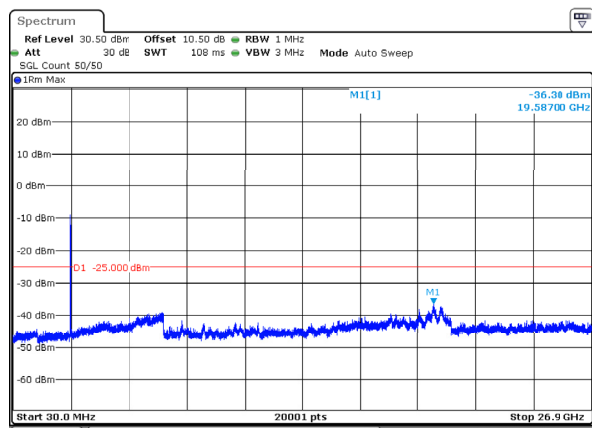
n41_50MHz_30kHz_2664.99MHz_DFT-s-OFDM QPSK_RB128@0 -36.30dBm
