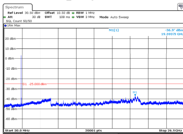
n41_90MHz_30kHz_2592.99MHz_DFT-s-OFDM QPSK_RB1@0 -36.97dBm
