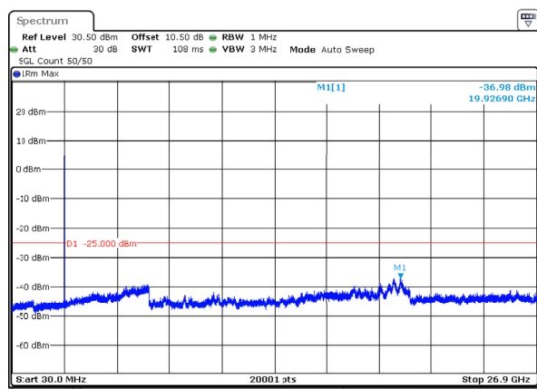
n41_30MHz_30kHz_2674.98MHz_DFT-s-OFDM QPSK_RB1@77 -36.98dBm
