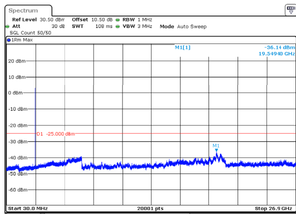
n41_30MHz_30kHz_2674.98MHz_DFT-s-OFDM QPSK_RB1@0 -36.14dBm
