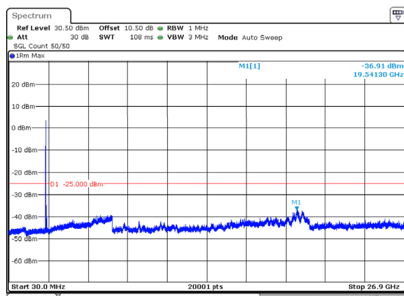
n41_90MHz_30kHz_2541MHz_DFT-s-OFDM QPSK_RB1@0 -36.91dBm
