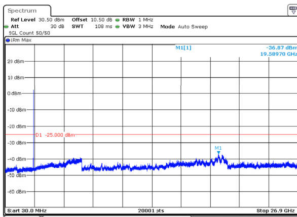
n41_20MHz_30kHz_2592.99MHz_DFT-s-OFDM QPSK_RB1@50 -36.87dBm
