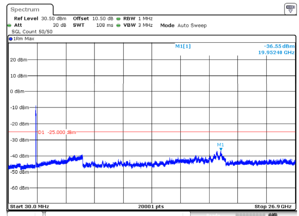
n41_60MHz_30kHz_2592.99MHz_DFT-s-OFDM QPSK_RB162@0 -36.55dBm
