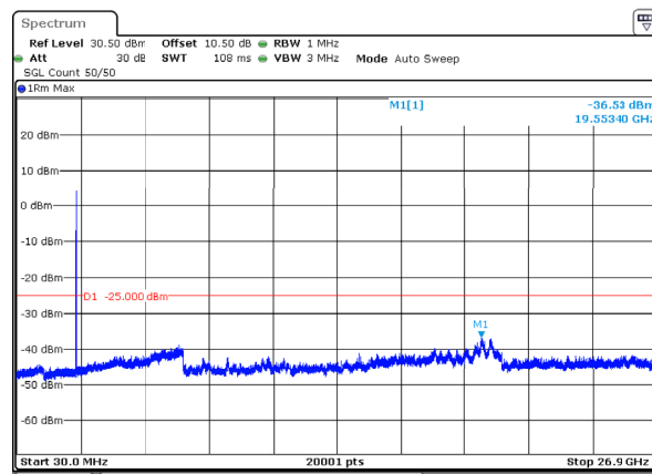
n41_30MHz_30kHz_2511MHz_DFT-s-OFDM QPSK_RB1@0 -36.53dBm
