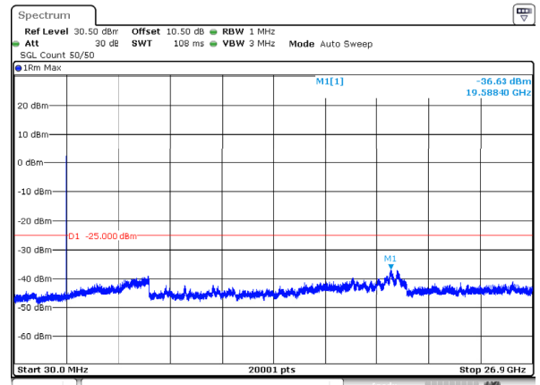
n41_15MHz_30kHz_2682.48MHz_DFT-s-OFDM QPSK_RB1@0 -36.63dBm
