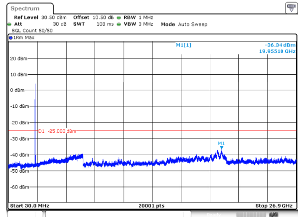
n41_60MHz_30kHz_2526MHz_DFT-s-OFDM QPSK_RB1@0 -36.34dBm
