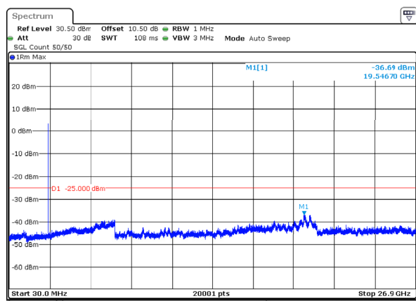
n41_50MHz_30kHz_2592.99MHz_DFT-s-OFDM QPSK_RB1@0 -36.69dBm
