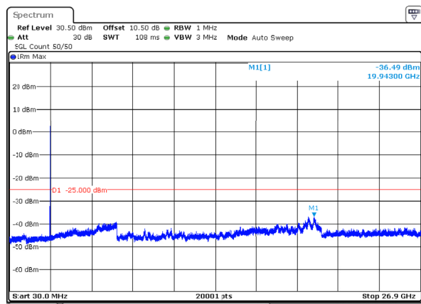
n41_60MHz_30kHz_2659.98MHz_DFT-s-OFDM QPSK_RB1@161 -36.49dBm
