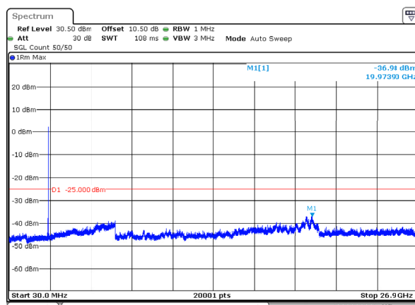
n41_90MHz_30kHz_2541MHz_DFT-s-OFDM QPSK_RB1@244 -36.98dBm
