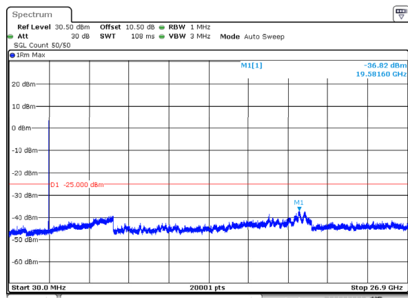
n41_40MHz_30kHz_2670MHz_DFT-s-OFDM QPSK_RB1@105 -36.82dBm
