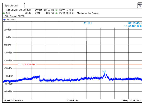
n41_80MHz_30kHz_2649.99MHz_DFT-s-OFDM QPSK_RB1@216 -37.19dBm
