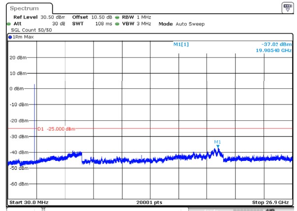
n41_20MHz_30kHz_2506.02MHz_DFT-s-OFDM QPSK_RB1@50 -37.02dBm
