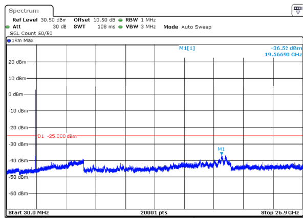
n41_30MHz_30kHz_2592.99MHz_DFT-s-OFDM QPSK_RB1@77 -36.52dBm
