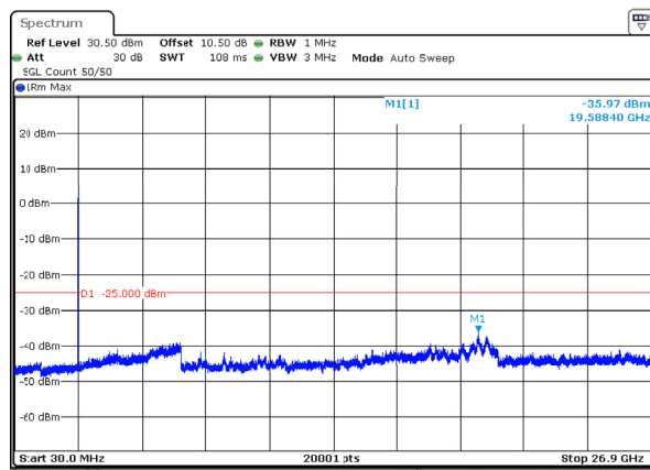
n41_20MHz_30kHz_2679.99MHz_DFT-s-OFDM QPSK_RB1@0 -35.97dBm
