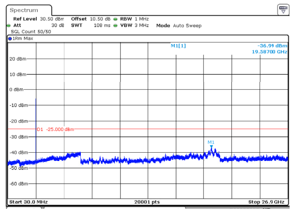
n41_15MHz_30kHz_2682.48MHz_DFT-s-OFDM QPSK_RB36@0 -36.99dBm
