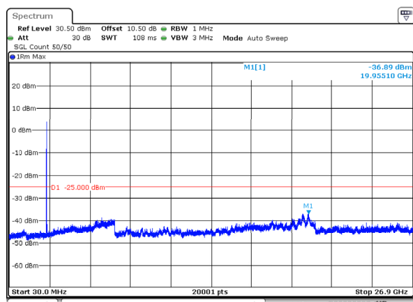
n41_50MHz_30kHz_2521.02MHz_DFT-s-OFDM QPSK_RB1@0 -36.89dBm
