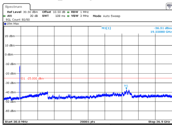
n41_90MHz_30kHz_2541MHz_DFT-s-OFDM QPSK_RB243@0 -36.51dBm
