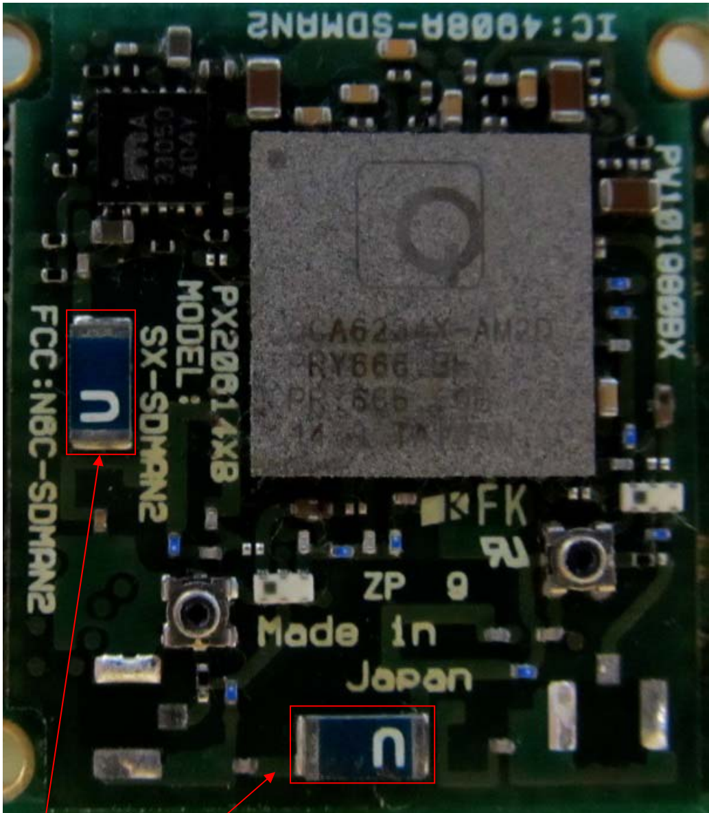
Antenna
