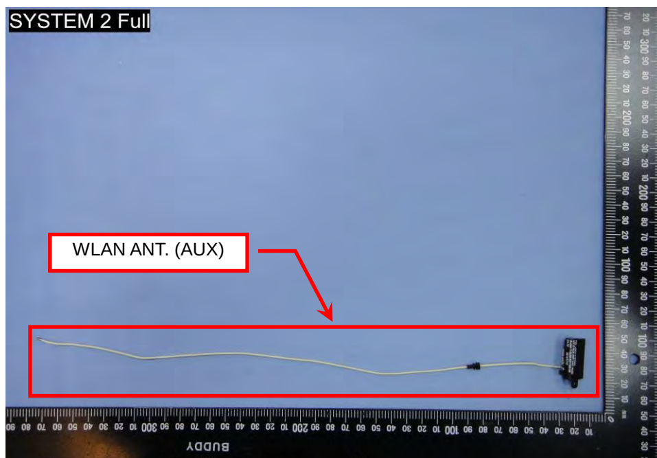
EUT Photo (196)
