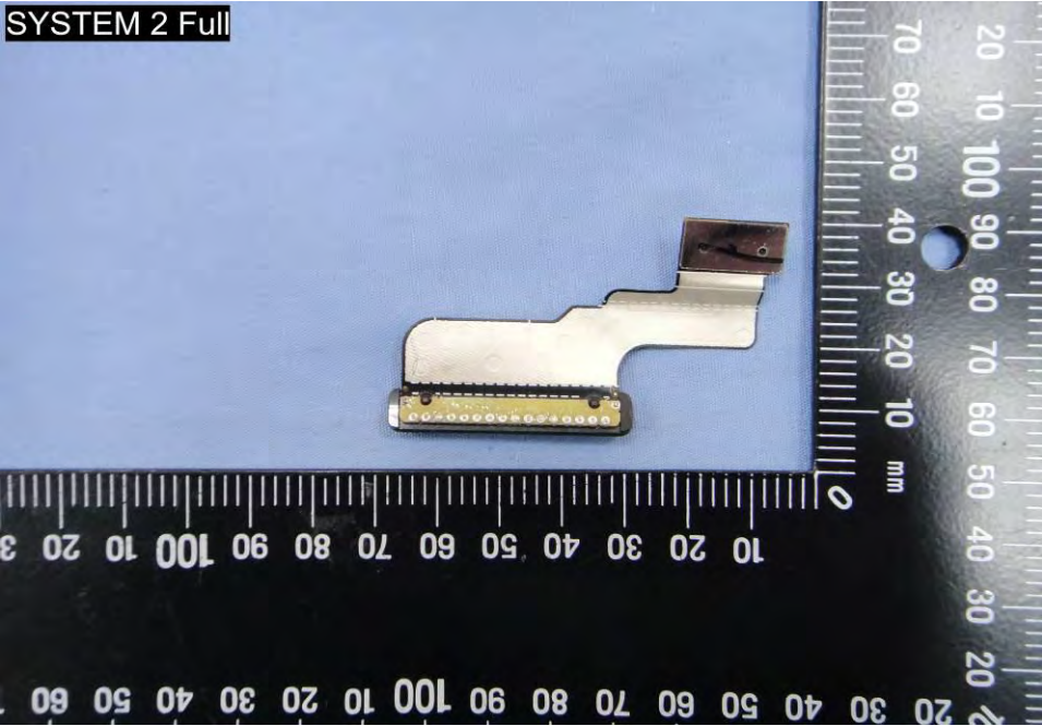
EUT Photo (178)
