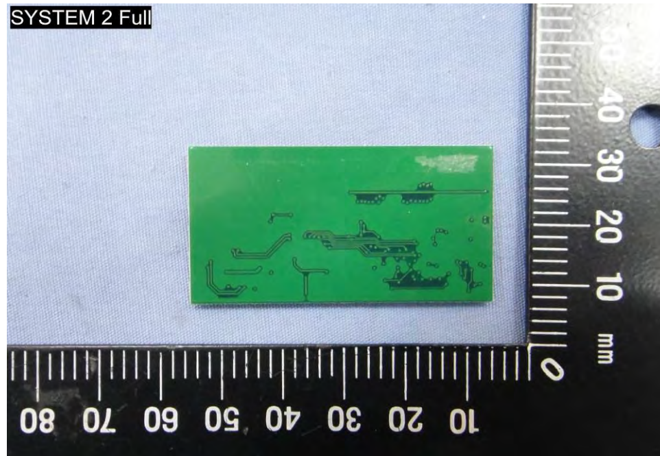
EUT Photo (214)
