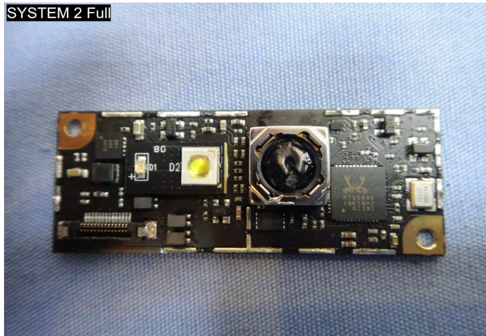
EUT Photo (170)
