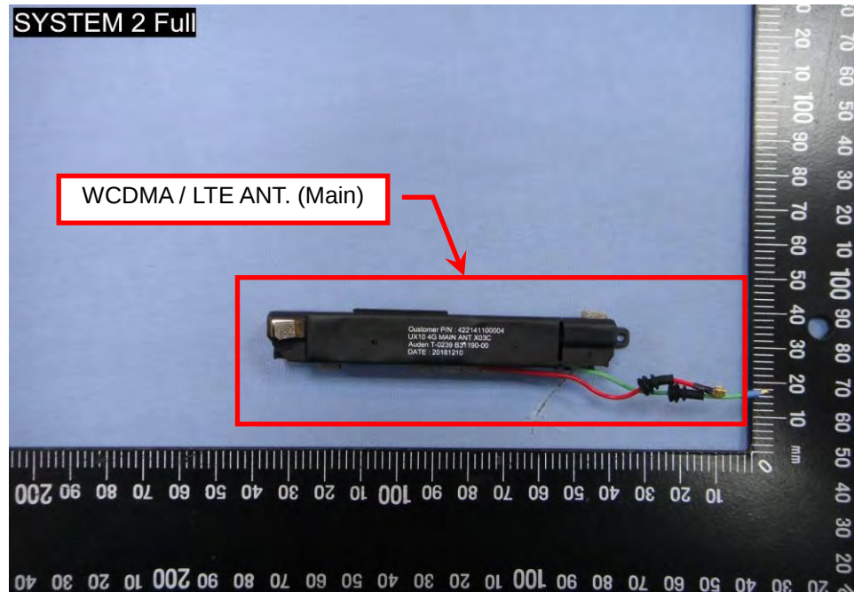
EUT Photo (186)
