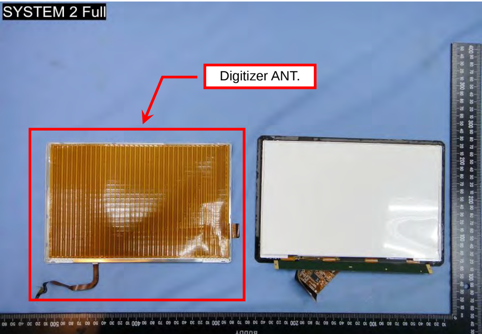
EUT Photo (220)
