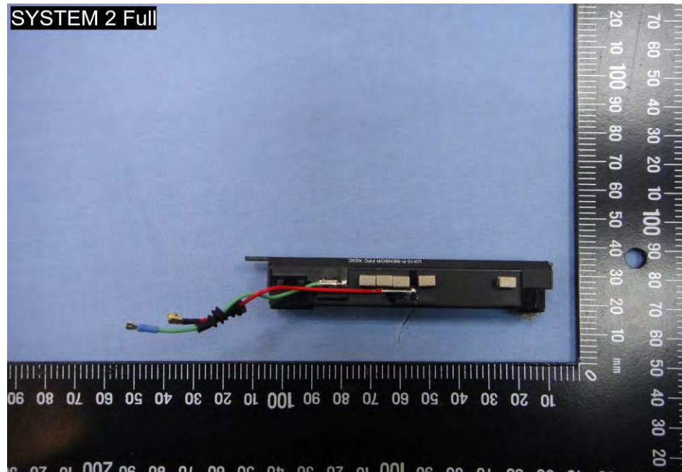
EUT Photo (188)
