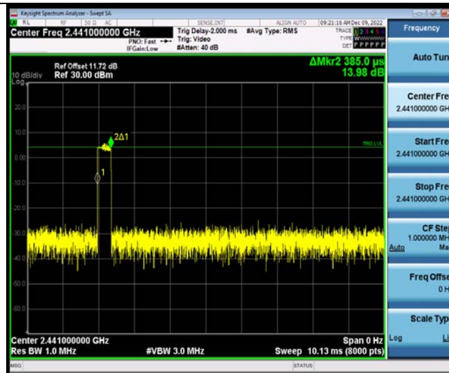
3DH3_Ant1_Hop
