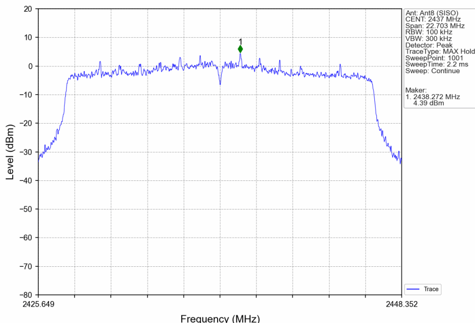
802.11ax(HEW20)_MCH_2437MHz_SU_/_Ant8 (SISO)_NTNV
