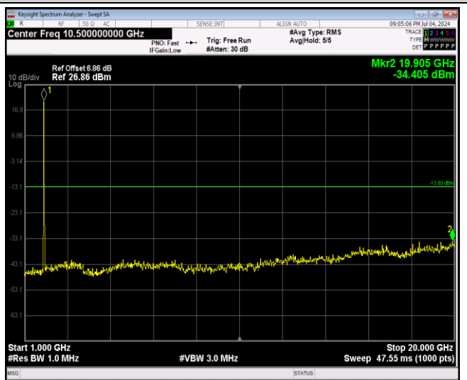
Band25-20MHz-QPSK-26140-1RB#0-Range2:1000~ 20000MHz
