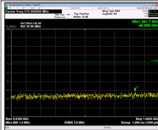
Band25-20MHz-QPSK-26140-1RB#0-Range1:30~1 000MHz
