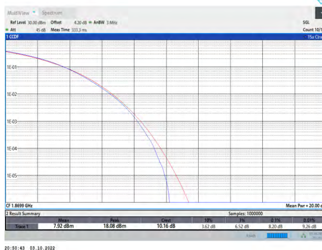
2-2-20MHz-20MHz-QPSK-QPSK-18801-18999-100RB#0-100RB#0
