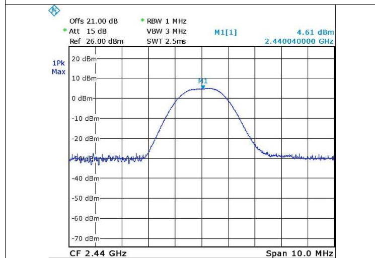
Figure 12. 2440.0 MHz, BLE
