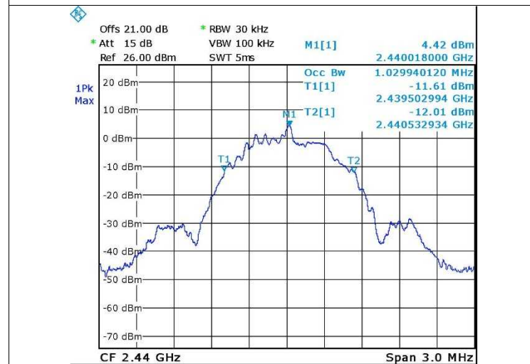
Figure 17. 2440.0 MHz, BLE
