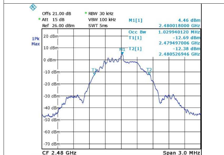
Figure 18. 2480.0 MHz, BLE
