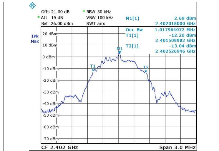
Figure 16. 2402.0 MHz, BLE
