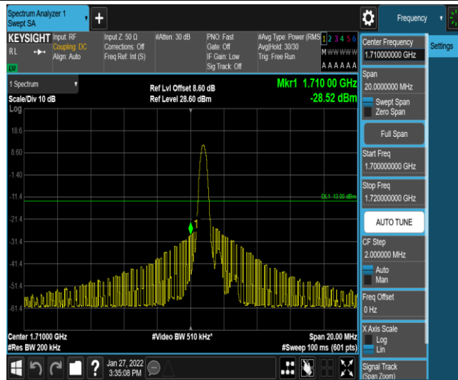
Band4-10MHz-QPSK-20000-1-0-Low--28.52-PASS
