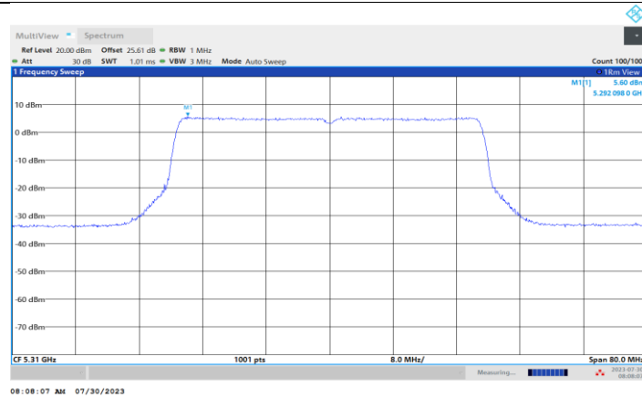
11BE40MIMO_Ant1_5310
