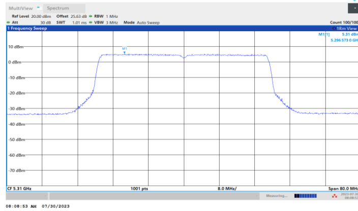
11BE40MIMO_Ant2_5310
