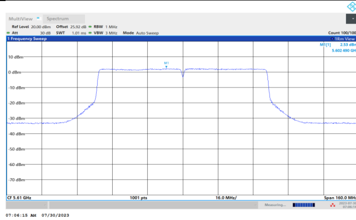
11AC80MIMO_Ant2_5610
