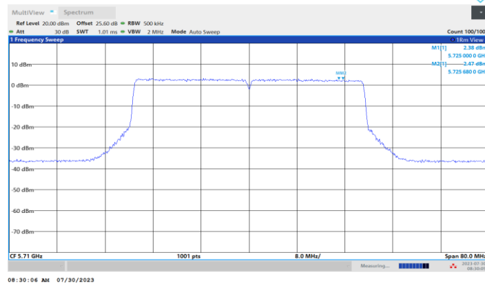
11BE40MIMO_Ant2_5710_UNII-3
