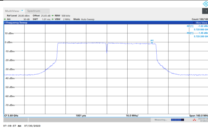
11AC80MIMO_Ant2_5690_UNII-3
