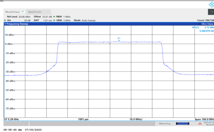
11BE80MIMO_Ant1_5290
