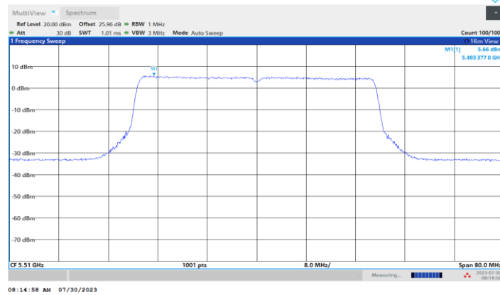
11BE40MIMO_Ant1_5510
