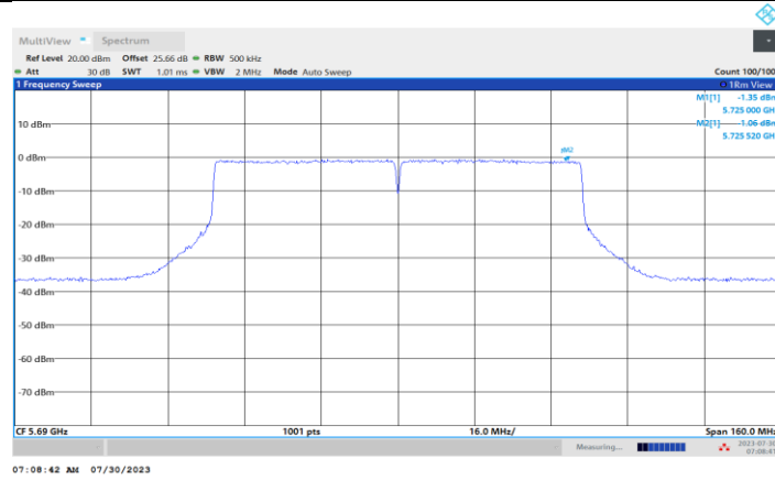
11AC80MIMO_Ant1_5690_UNII-3
