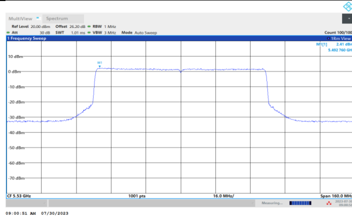
11BE80MIMO_Ant1_5530
