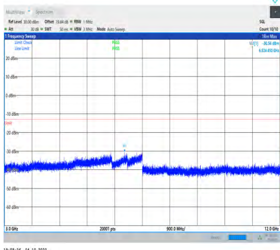
1-N25-PC3-15-40-L-1-DFT-QPSK-Inner_1RB_Left-1 @1-3000-12000-Ant1-6924.45--30.56--13-PASS
