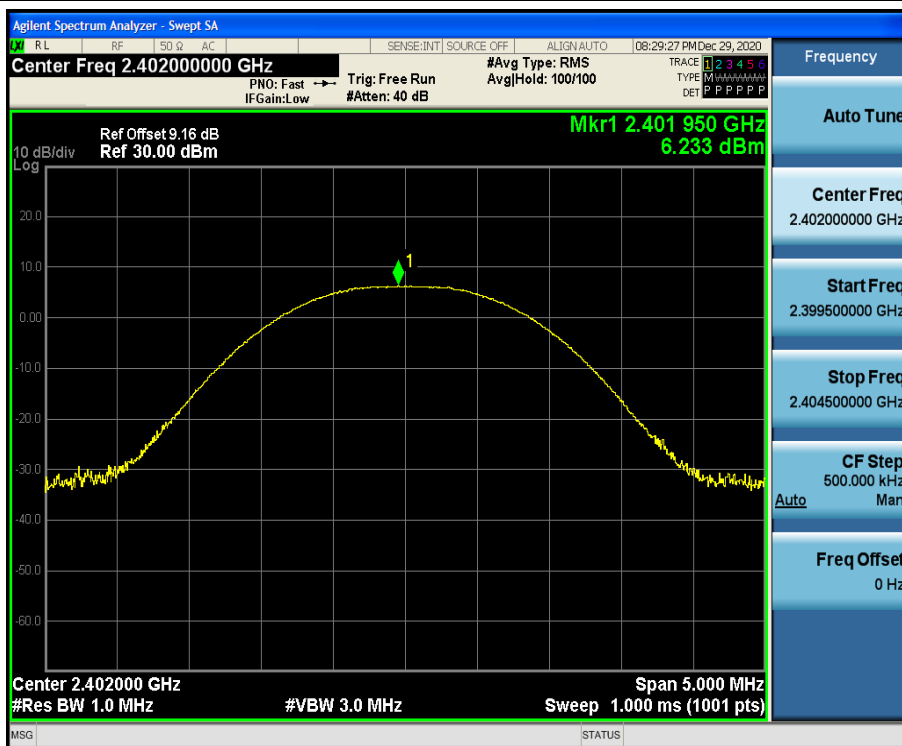
GFSK mode-CH00
