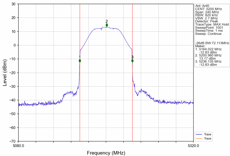
80M_MCH_5200MHz_Ant0_NTNV
