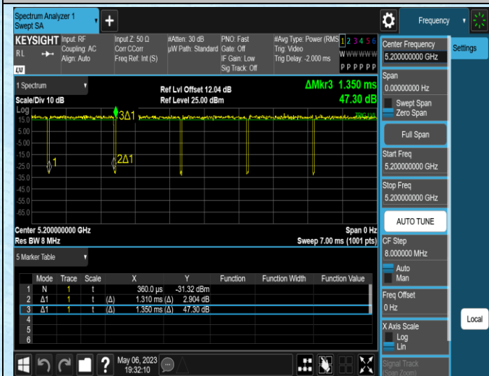
NTNV-11N20MIMO-Ant1-5200
