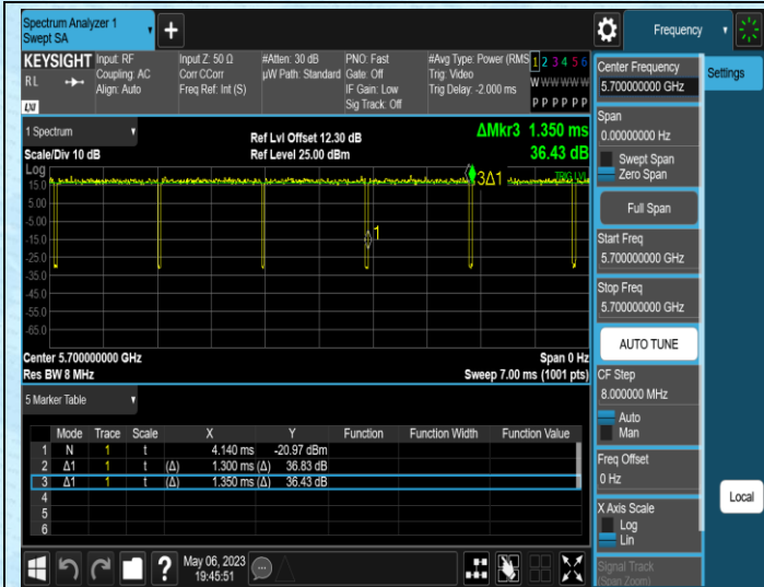
NTNV-11N20MIMO-Ant1-5700
