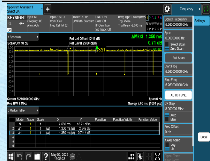
NTNV-11N20MIMO-Ant1-5260
