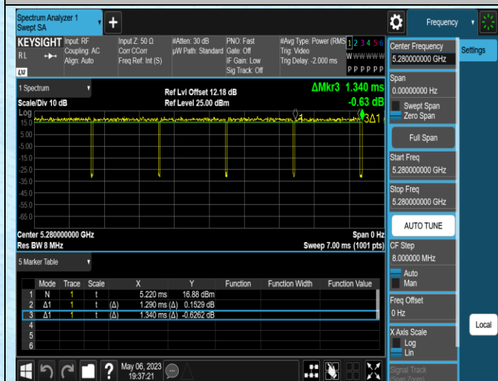
NTNV-11N20MIMO-Ant1-5280
