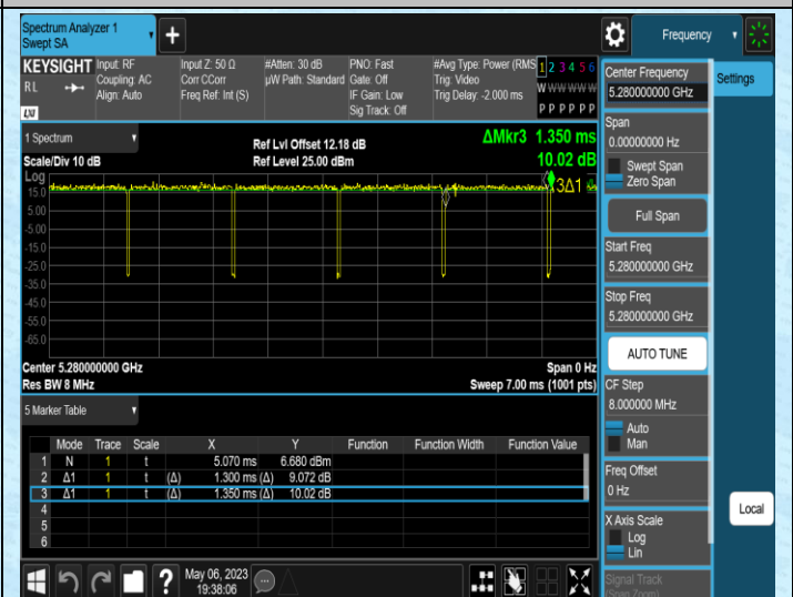
NTNV-11N20MIMO-Ant2-5280
