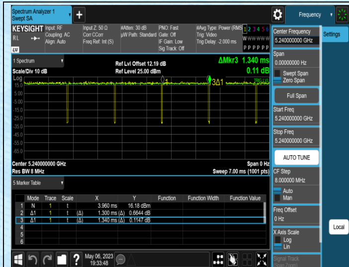
NTNV-11N20MIMO-Ant1-5240
