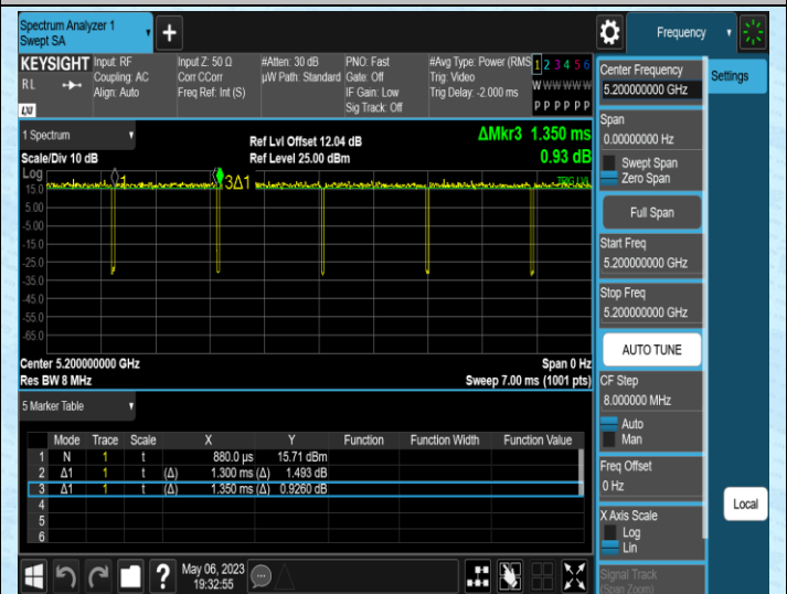
NTNV-11N20MIMO-Ant2-5200
