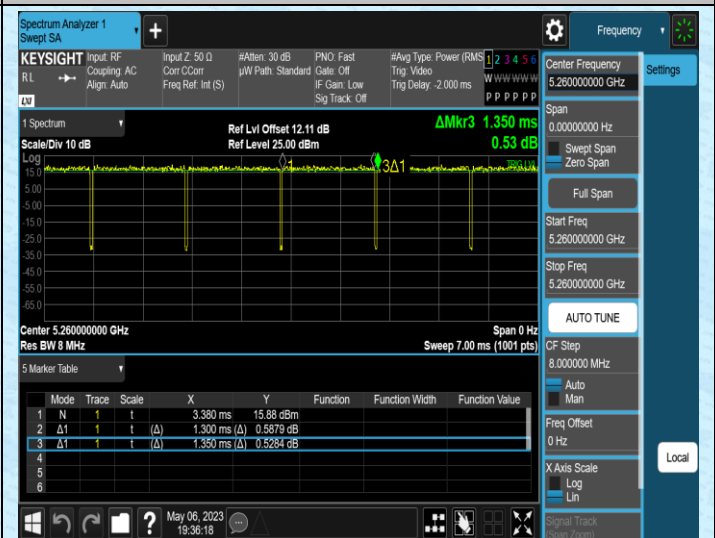
NTNV-11N20MIMO-Ant2-5260
