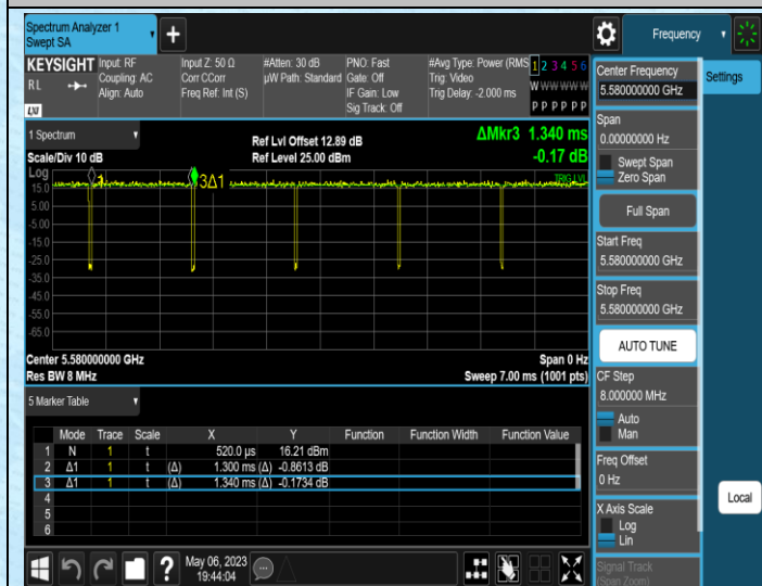
NTNV-11N20MIMO-Ant1-5580
