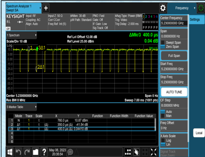
NTNV-11AC40MIMO-Ant1-5230
