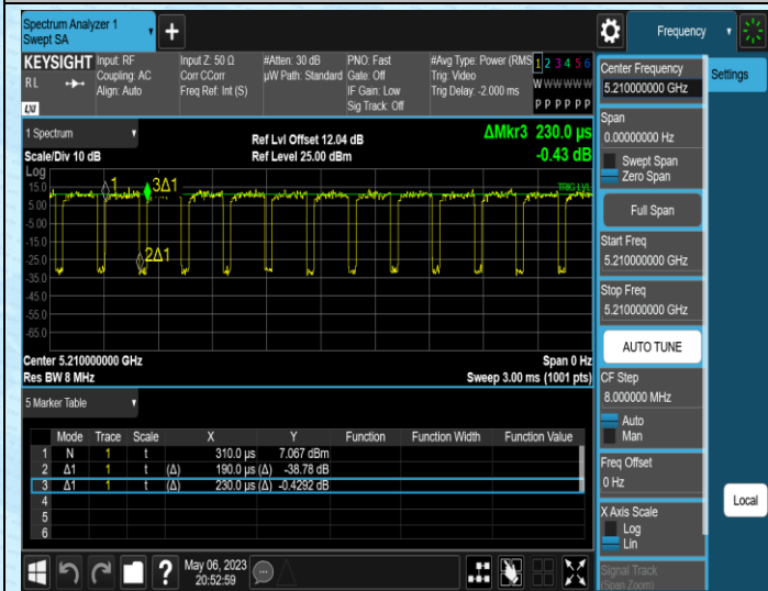
NTNV-11AC80MIMO-Ant1-5210
