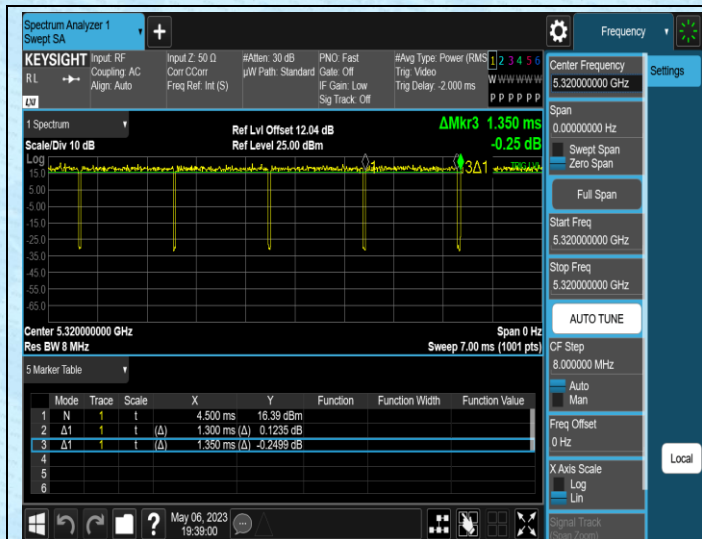
NTNV-11N20MIMO-Ant1-5320
