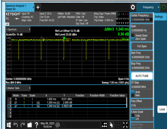
NTNV-11N20MIMO-Ant1-5500
