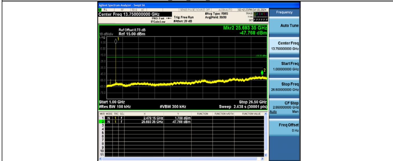
GFSK_Ant1_2478_1000~26500
