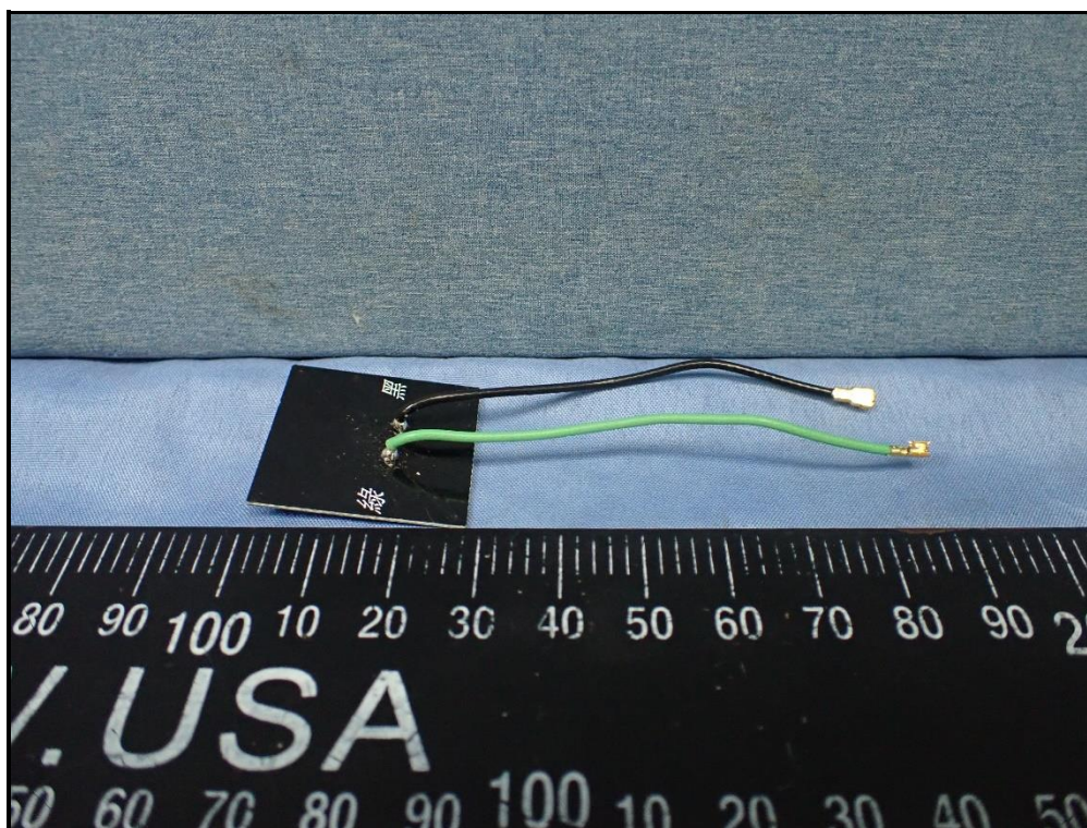
2GA Antenna
