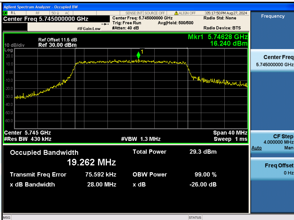
11AX20MIMO-Ant3-5745
