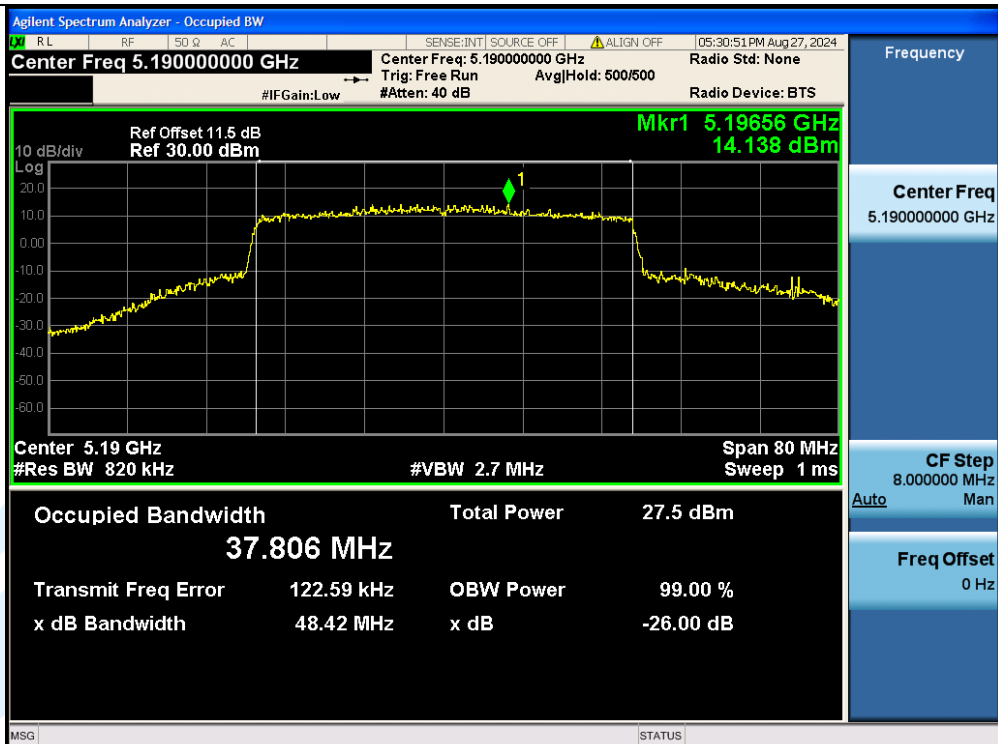
11AX40MIMO-Ant3-5190
