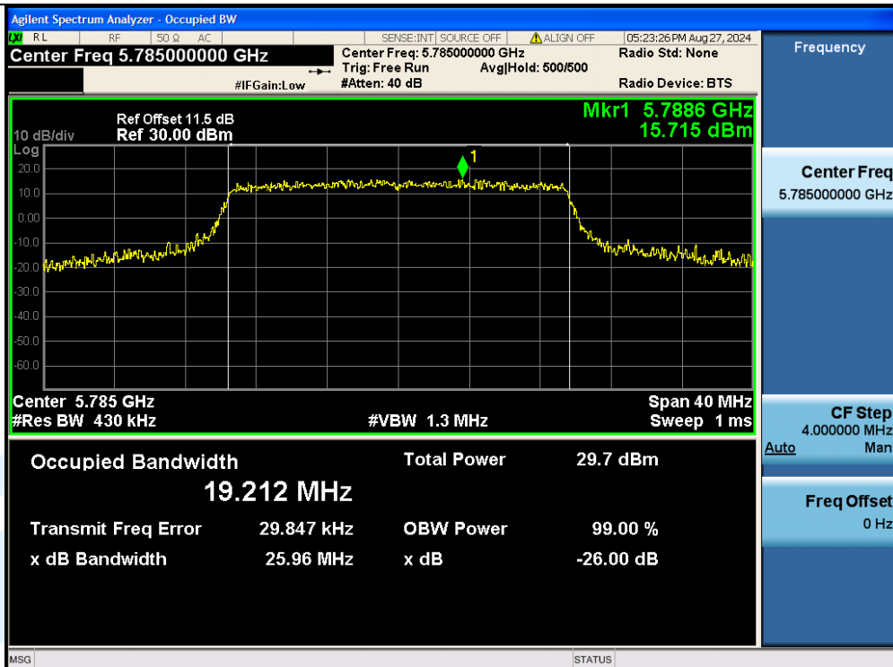
11AX20MIMO-Ant3-5785
