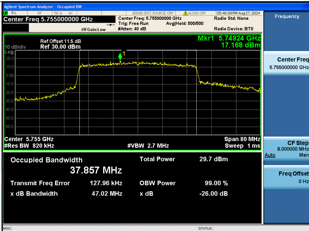
11AX40MIMO-Ant3-5755
