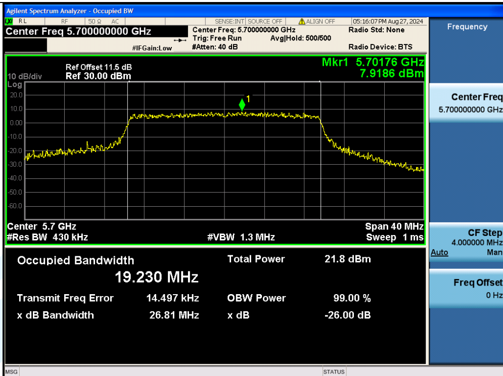
11AX20MIMO-Ant3-5700
