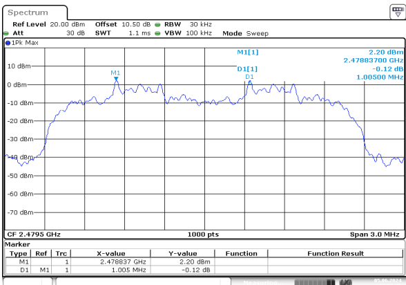
\pi/4 -DQPSK_High
