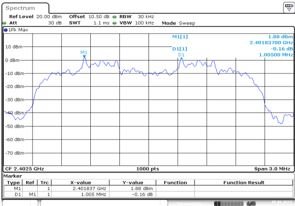
\pi/4 -DQPSK_Low
