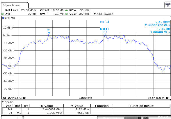
\pi/4 -DQPSK_Middle
