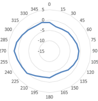
6525MHz-theta=90
