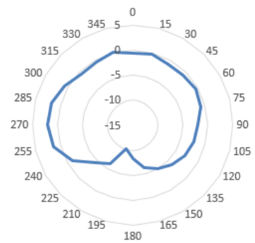
6925MHz-theta=90
