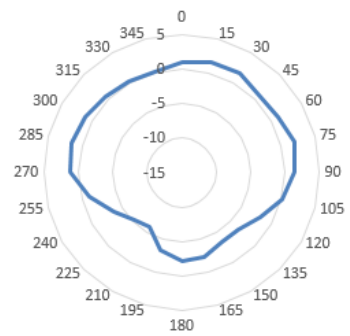
6925MHz-theta=90
