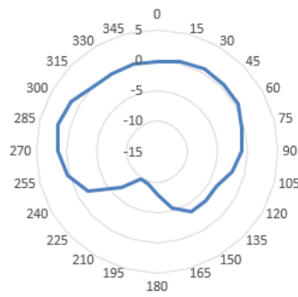
6125MHz-theta=90
