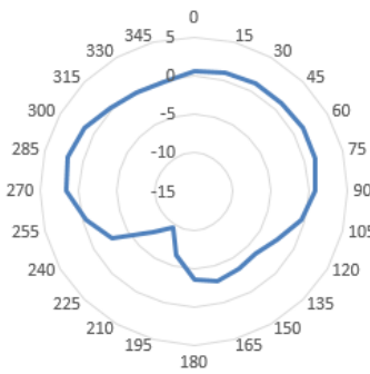
6525MHz-theta=90
