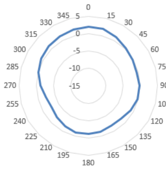
6125MHz-theta=90
