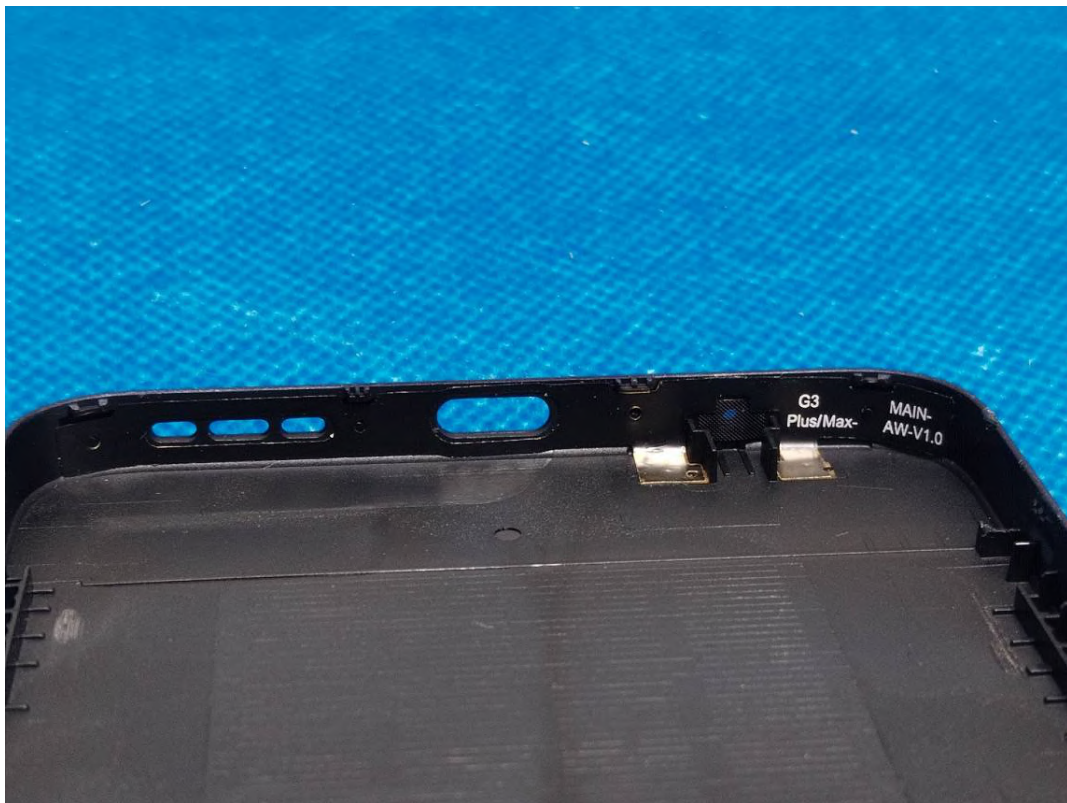
WWAN Main Antenna(GSM850, WCDMA B5,LTE B5/B7/B12/B41)
