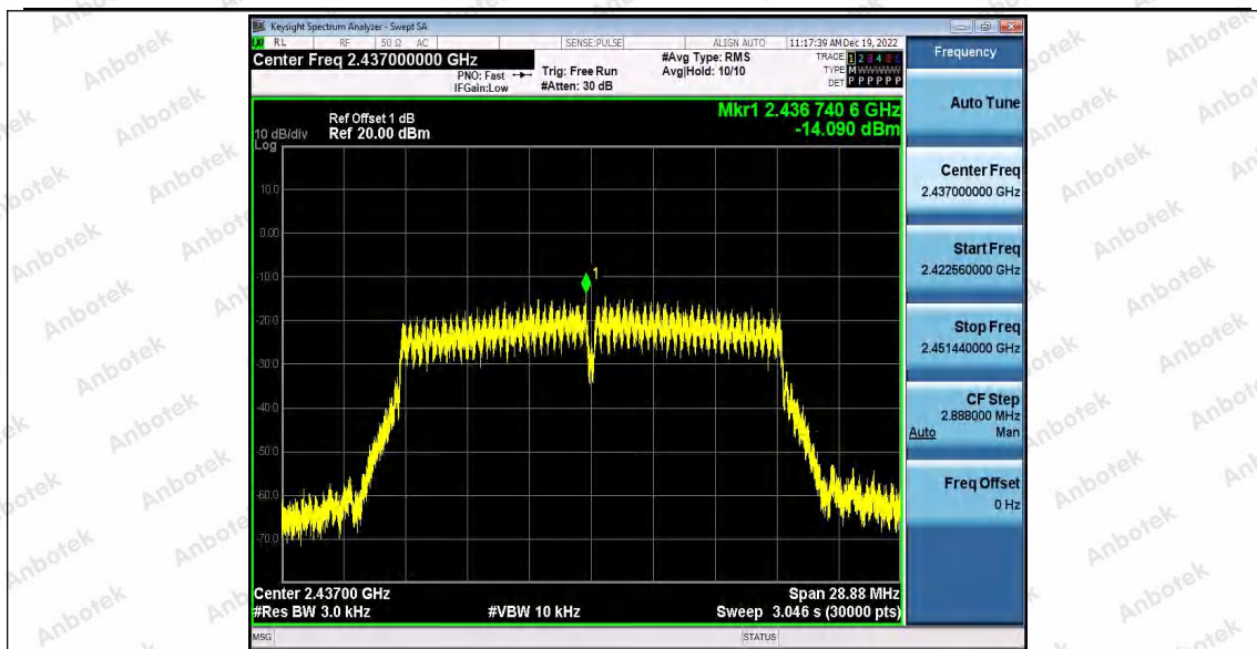
11N20_Ant2_2437
