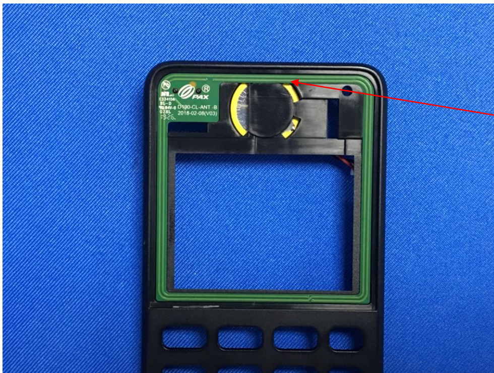
NFC antenna
