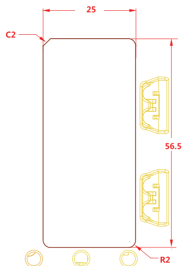
尺寸图
