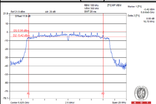
802.11n (20MHz)
