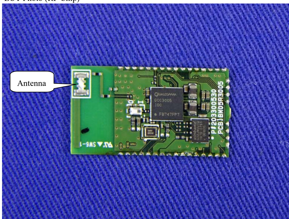
(10) EUT Photo (RF Chip)
