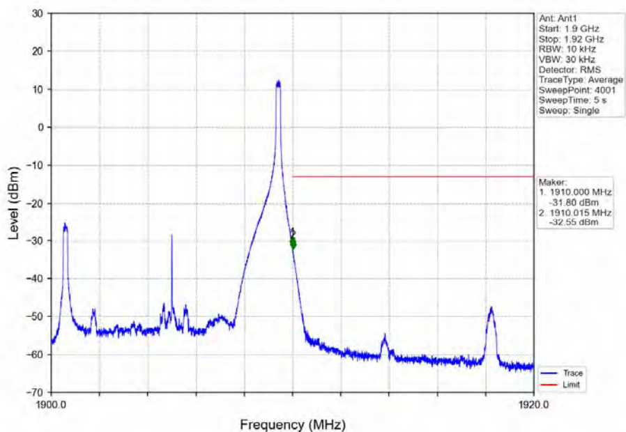
Band2_10MHz_QPSK_HCH_1905MHz_RB_1_49_NTNV
