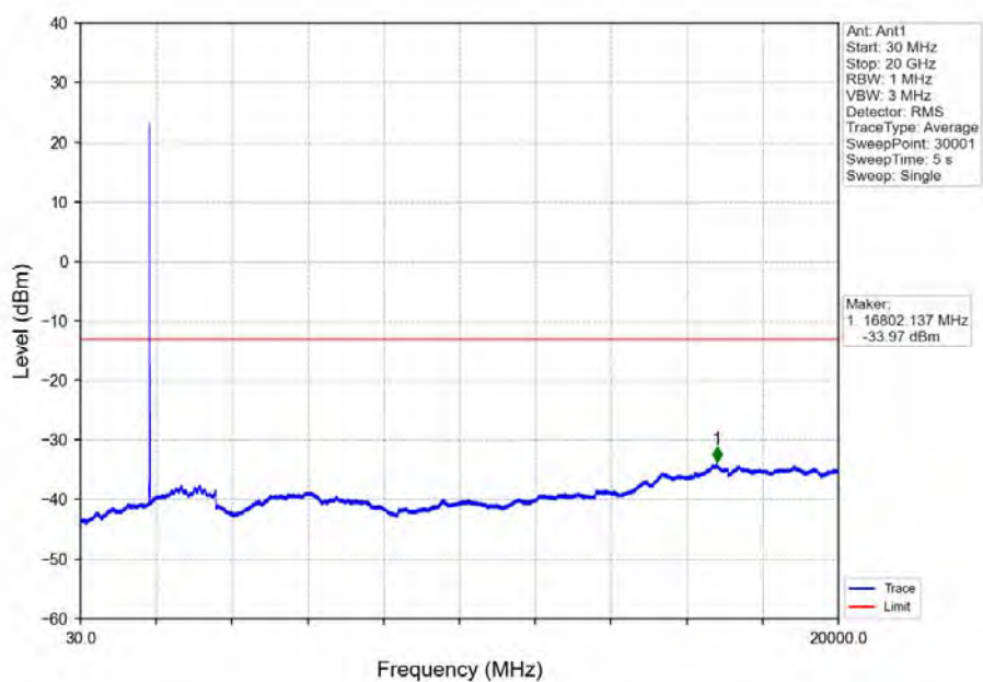
Band2_10MHz_16QAM_LCH_1855MHz_RB_50_0_NTNV
