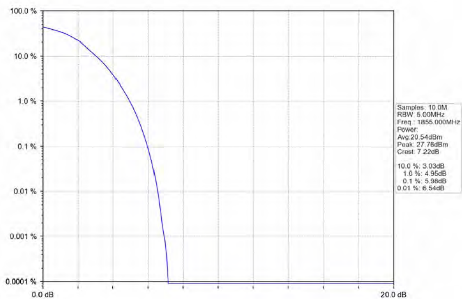
Band2_10MHz_16QAM_LCH_1855MHz_RB_50_0_NTNV
