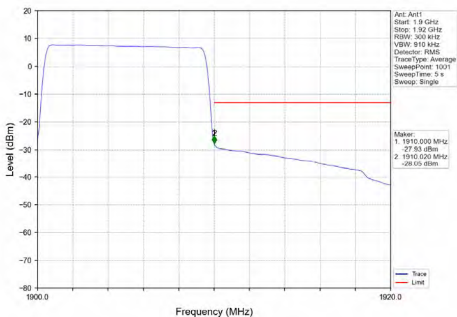
Band2_10MHz_16QAM_HCH_1905MHz_RB_50_0_NTNV
