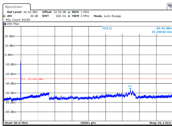
n38_30MHz_30kHz_2595MHz_DFT-s-OFDM QPSK_RB75@0 -36.55dBm
