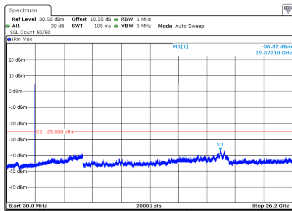
n38_30MHz_30kHz_2585MHz_DFT-s-OFDM QPSK_RB1@0 -36.82dBm
