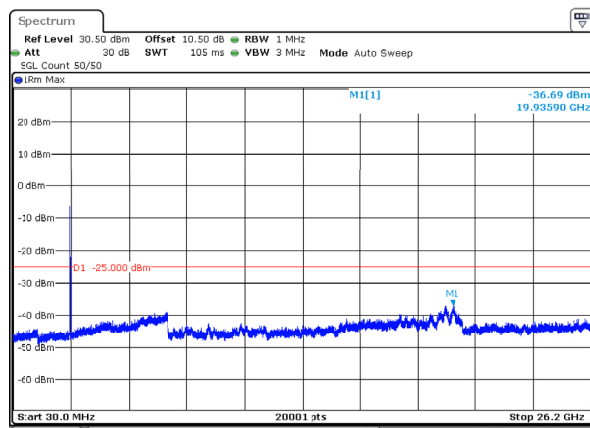
n38_30MHz_30kHz_2585MHz_DFT-s-OFDM QPSK_RB75@0 -36.69dBm
