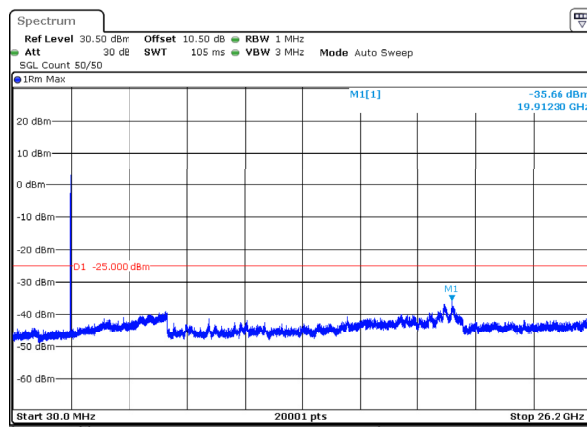
n38_30MHz_30kHz_2585MHz_DFT-s-OFDM QPSK_RB1@77 -35.66dBm
