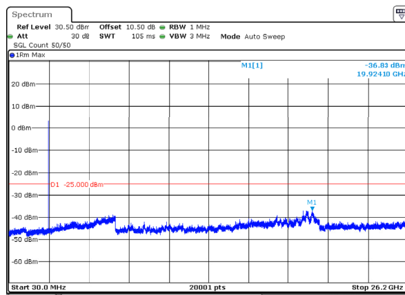
n38_30MHz_30kHz_2595MHz_DFT-s-OFDM QPSK_RB1@0 -36.83dBm
