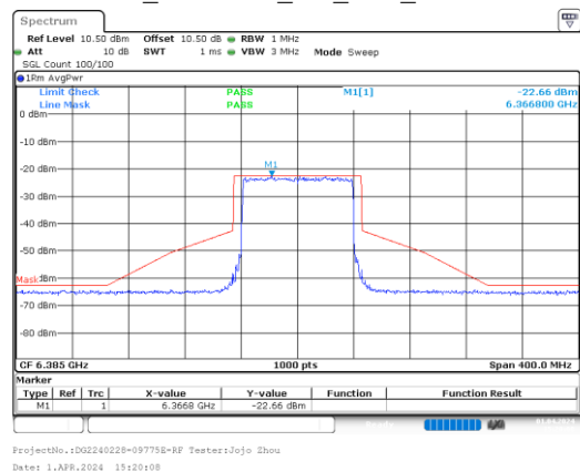
ax80_6385MHz_RU_26/0_Chain 0
