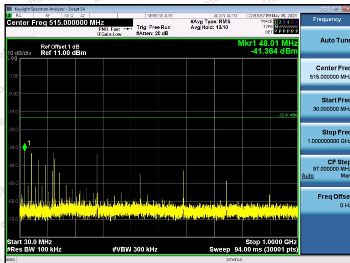
2.4G-Ant1-2408-30~1000-PASS
