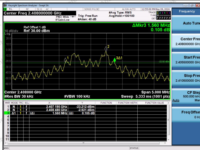
2.4G-Ant1-2408
