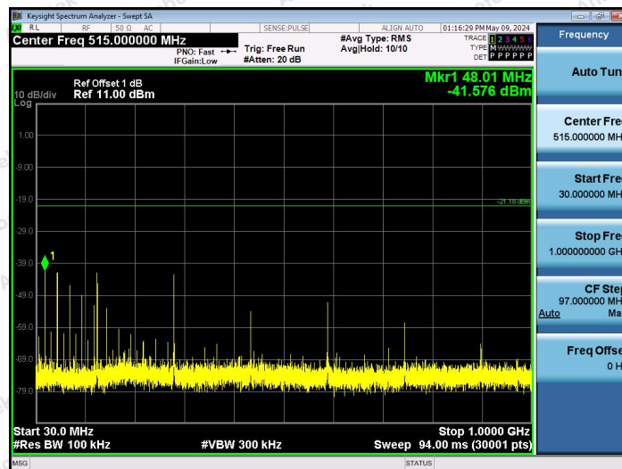
2.4G-Ant1-2474-30~1000-PASS
