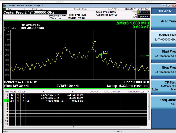
2.4G-Ant1-2474
