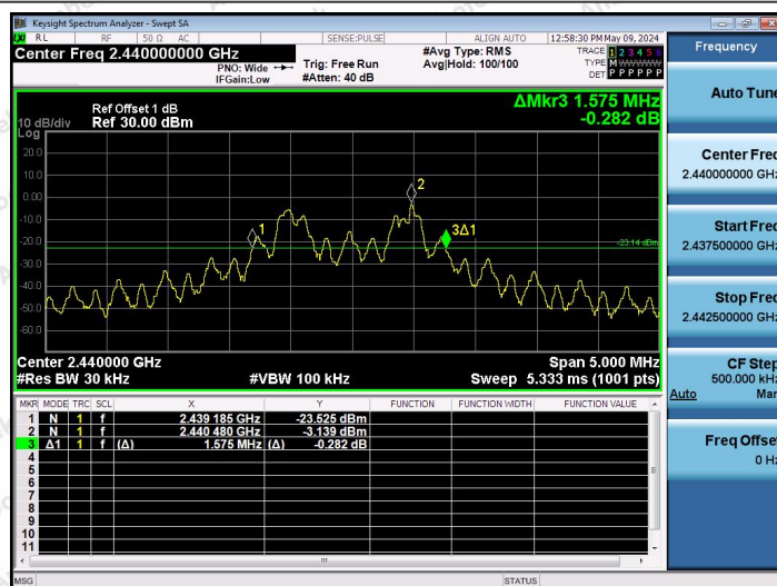
2.4G-Ant1-2440
