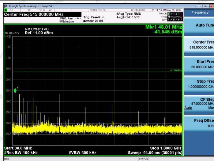
2.4G-Ant1-2440-30~1000-PASS
