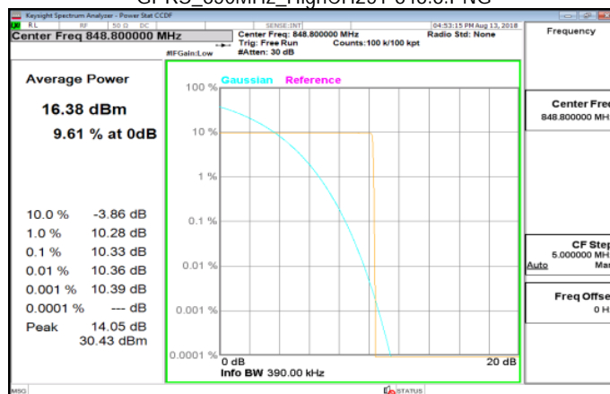
GPRS_850MHz_HighCH251-848.8.PNG
