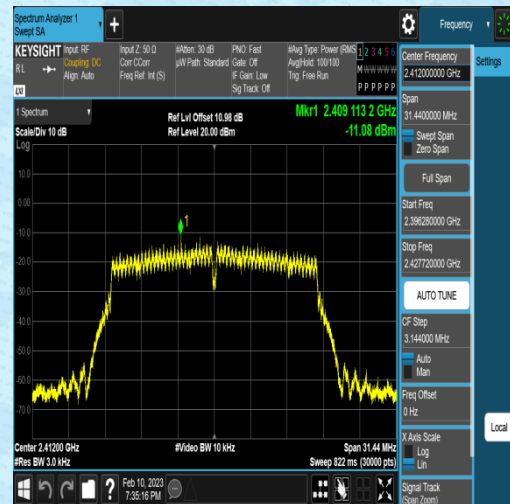
11N20MIMO-Ant2-2412--11.08-0.00-0.00-0.00
