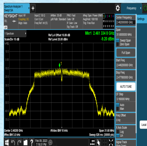
11G-Ant1-2462--9.20-0.00-0.00-0.00
