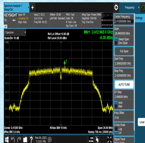
11G-Ant1-2412--8.38-0.00-0.00-0.00
