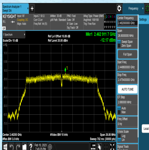
11N20MIMO-Ant1-2462--12.17-0.00-0.00-0.00
