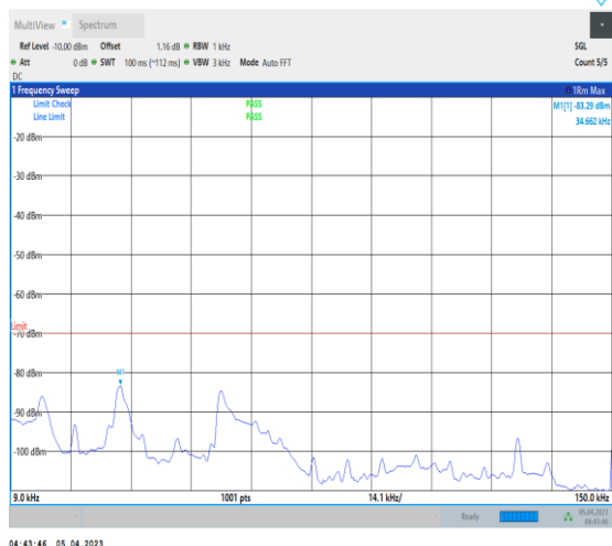
1-N48-PC3-30-40-L-1-DFT-PI2BPSK-Inner_1RB_Lef t-1@1-0.009-0.15-Ant0-0.02--83.29--70-PASS
