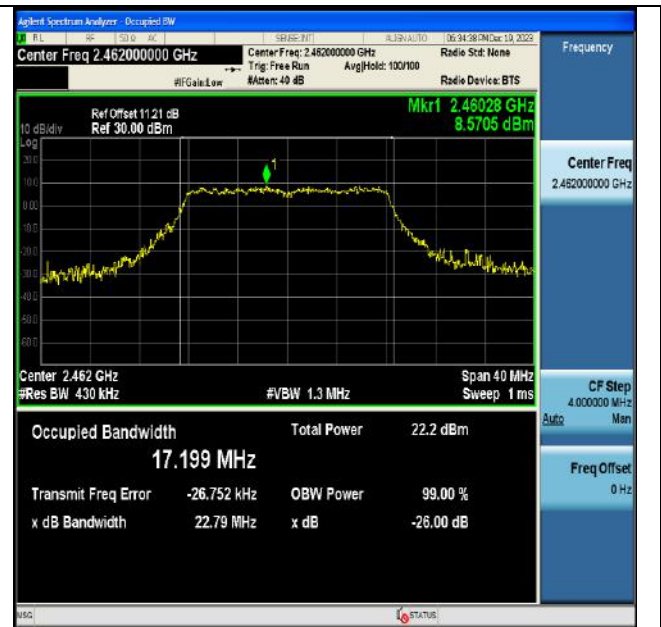
11G-Ant1-2462
