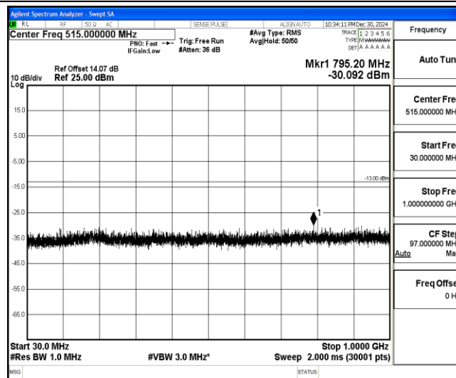
Band4-3MHz-QPSK-19965-1-0-Low-30-1000--30.09-PASS
