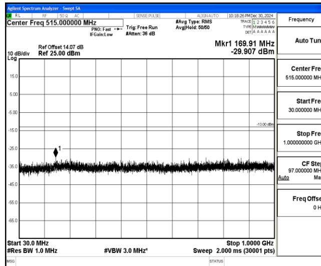
Band4-1.4MHz-16QAM-20175-1-0-Low-30-1000--29.91-PASS
