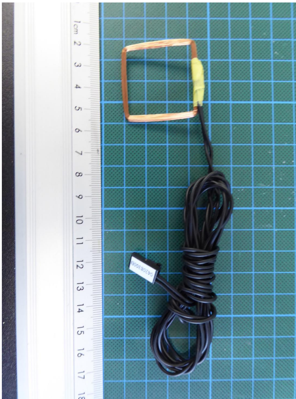
153615_11.JPG: Antenna 1 (0420830 0)
